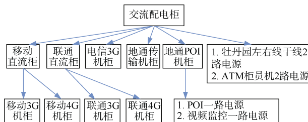
图 4 民用机房内配分布明细
