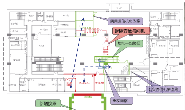
图 2 东侧站厅改造平面布置
