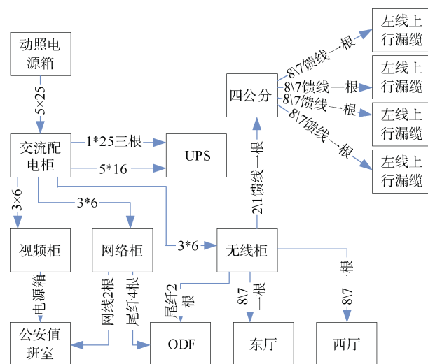
图 3 公安机房内配分布明细
