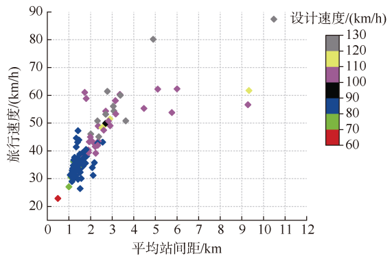
图 3 旅行速度和平均站间距的关系
