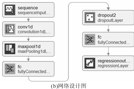
图3 一维CNN结构图与网络设计图
