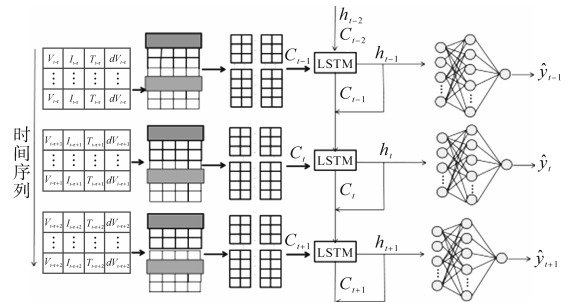
图4 CNN-LSTM结构图
