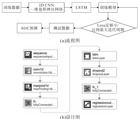
图5 CNN-LSTM网络流程图和设计图
