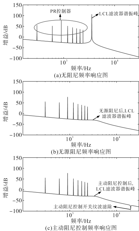
图5 系统的频率响应
