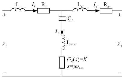
图3 带有主动阻尼装置的LCL滤波器的简化电路图
