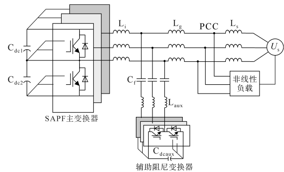
图1 SAPF系统框图
