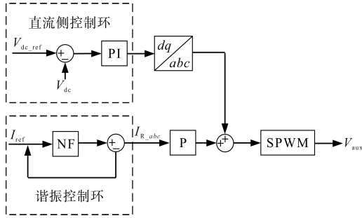
图2 主动阻尼变换器的控制算法
