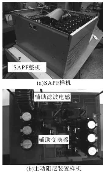
图6 实验样机图片
