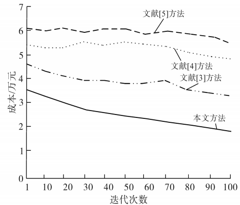
图4 不同方法的主动配电网选址定容网损成本
