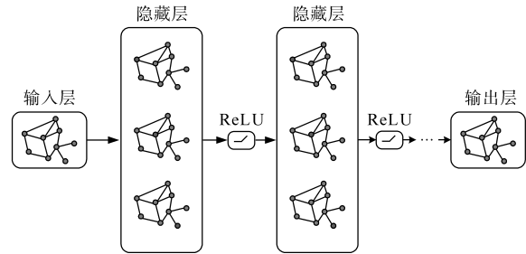
图2 图卷积神经网络结构图
