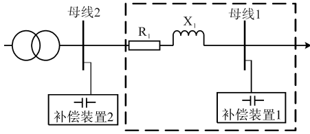
图1 项目边界示意图
