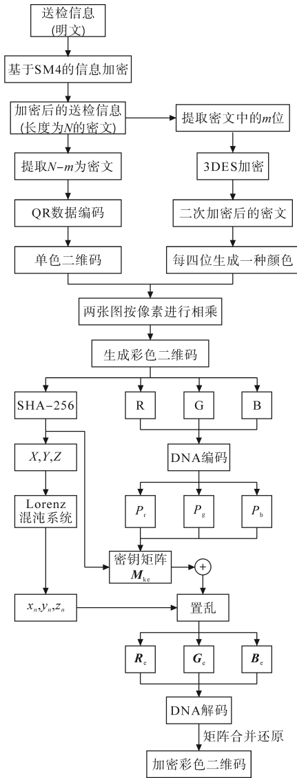
图2 加密流程图
