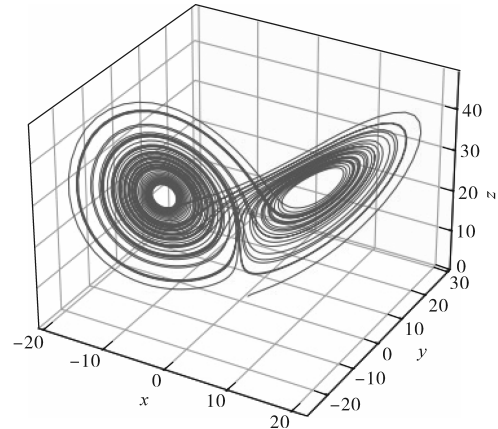
图3 Lorenz吸引子
