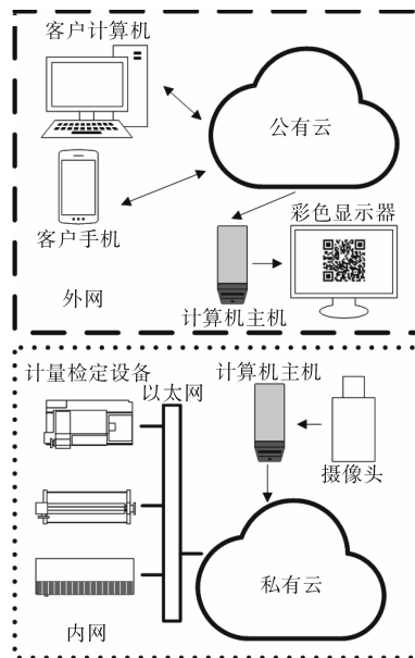
图1 基于加密二维码的电力计量物联网非电通信方法结构框图
