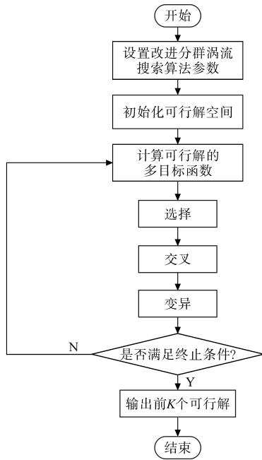
图1 改进分群涡流搜索算法生成初始解流程
