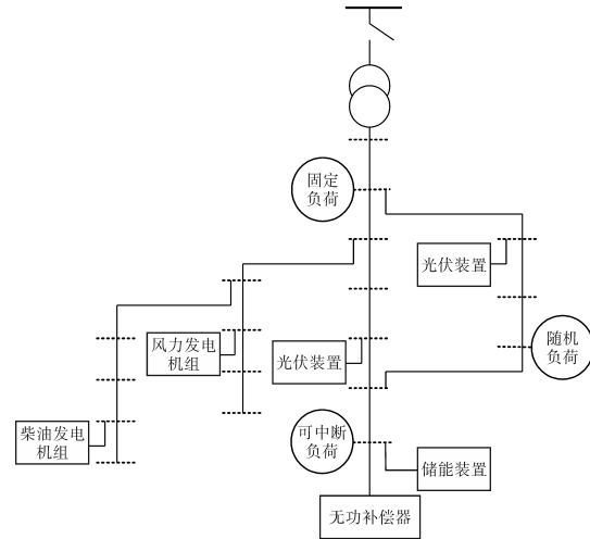
图2 IEEE 33节点配电网拓扑结构模型
