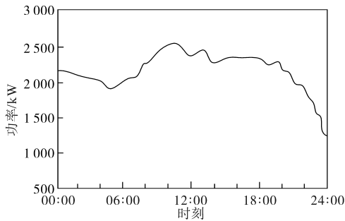
图3 配电网用电负荷需求变化曲线图
