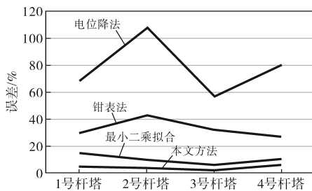
图9 杆塔接地电阻相对误差曲线
