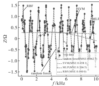
图10 神经网络拟合随机曲线结果
