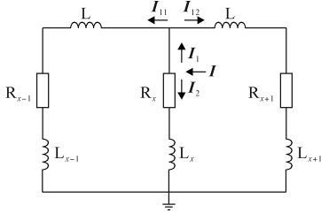
图4 杆塔接地电阻测量简化等效电路II
