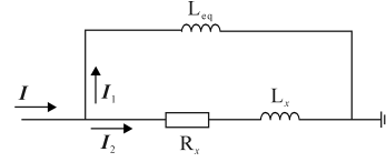
图5 杆塔接地电阻测量简化等效电路III
