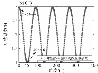
图8 四发射线圈和单接收线圈互感系数
