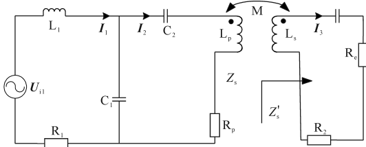
图5 化简等效电路模型
