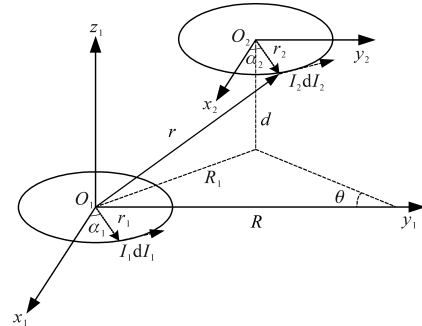
图2 单发射线圈与单接收线圈空间位置模型
