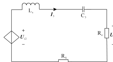
图7 二次侧等效模型
