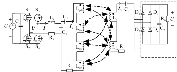
图4 系统电路模型
