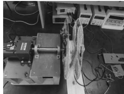
图12 四发射线圈与两接收线圈实验样机
