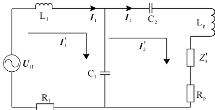
图6 二次侧折算到一次侧的等效模型
