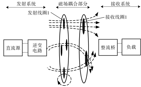
图1 平面旋转机构无线电能传输系统结构图
