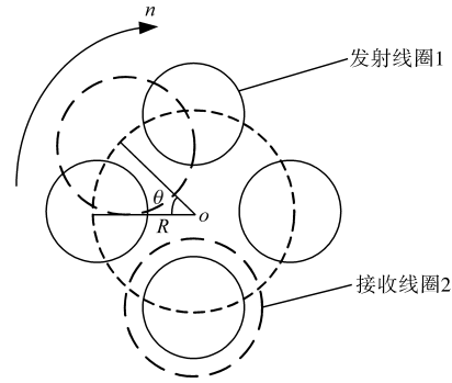
图3 四发射线圈与两接收线圈空间位置模型
