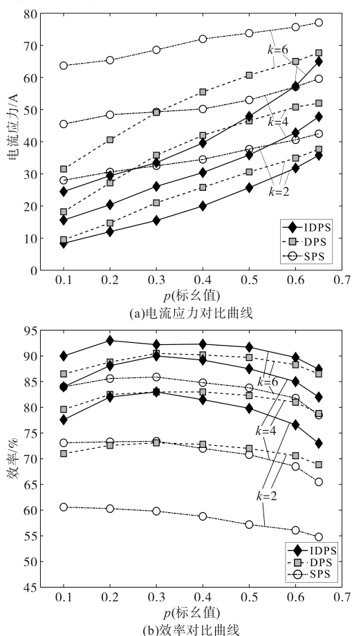
图7 不同电压传输比下的实验曲线
