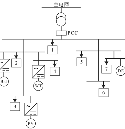
图9 微电网算例系统结构图
