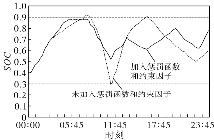
图12 SOC趋势对比图
