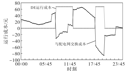
图14 全天微电网运行成本
