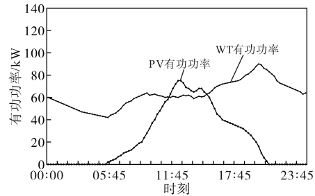
图10 光伏发电系统和风力发电系统全天有功功率输出
