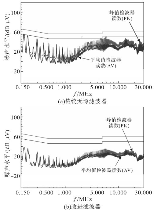
图10 车载充电机加入改进滤波器前、后传导电压法测试
