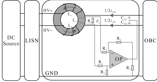
图3 混合 CSCI-EMI 滤波器的结构
