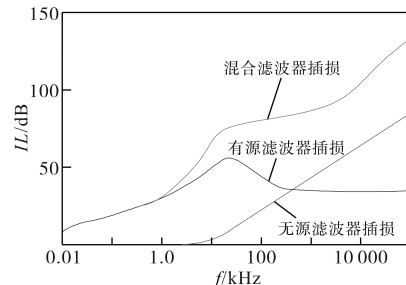
图6 混合滤波器及其组成部分的插损
