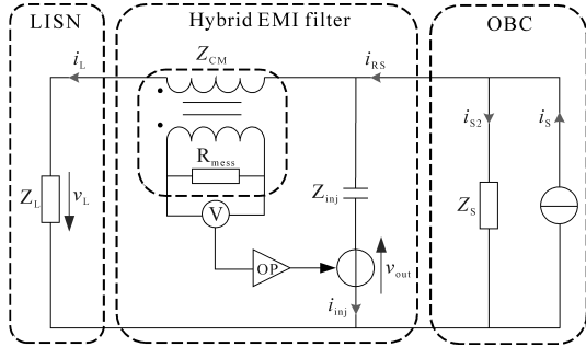
图4 混合 CSCI-EMI 滤波器等效电路
