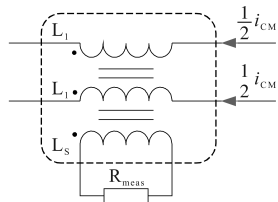
图7 带有附加传感绕组的共模扼流圈示意图
