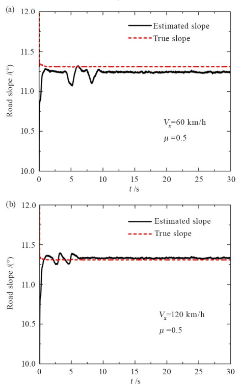
图 8 双移线工况( \mu = 0.5 )的定坡度(20%)估算结果:
