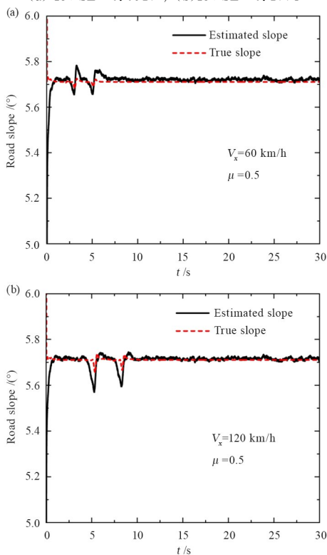
图 6 双移线工况( \mu = 0.5 )的定坡度(10%)估算结果:
