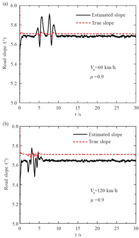
图 5 双移线工况( \mu = 0.9 )的定坡度(10%)估算结果:
