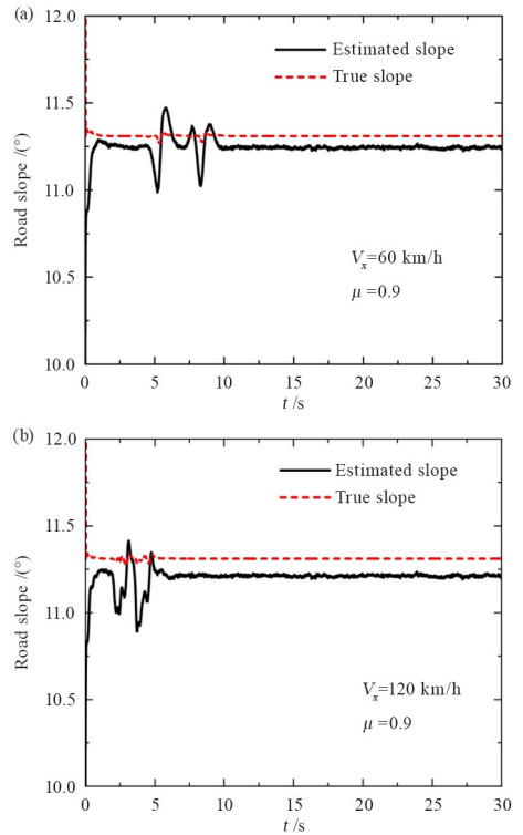
图 7 双移线工况( \mu = 0.9 )的定坡度(20%)估算结果:
