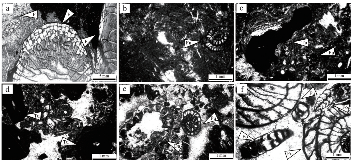
图7 窝托村珊瑚礁剖面的微相类型
