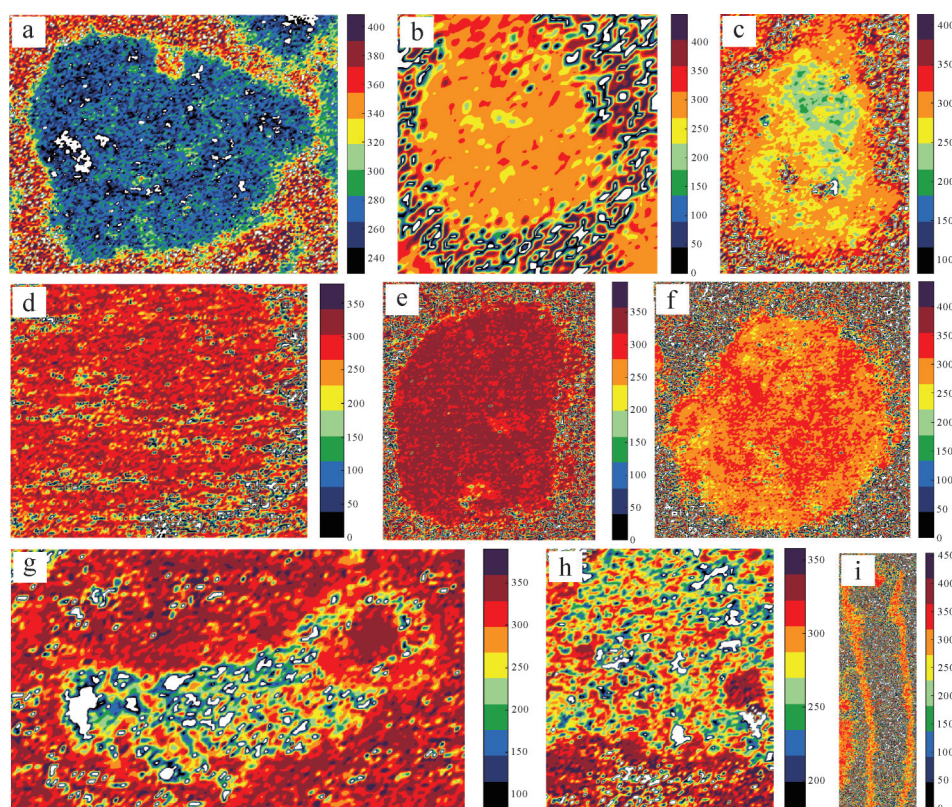
图 12 研究剖面的球粒、生物化石及介壳碎片外部泥晶套的拉曼温度平面分布图
