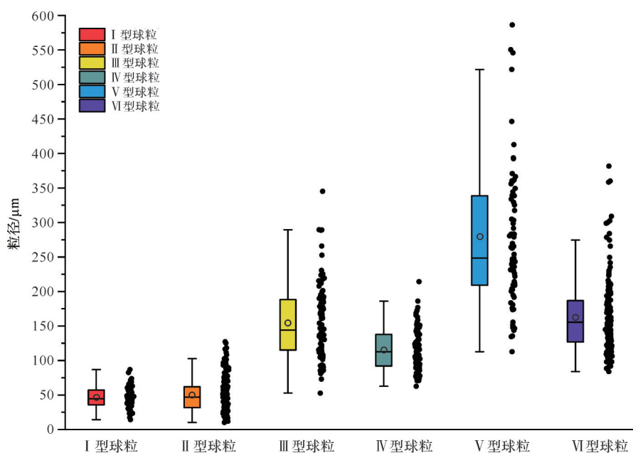
图7 不同类型球粒结构的粒径统计结果对比
