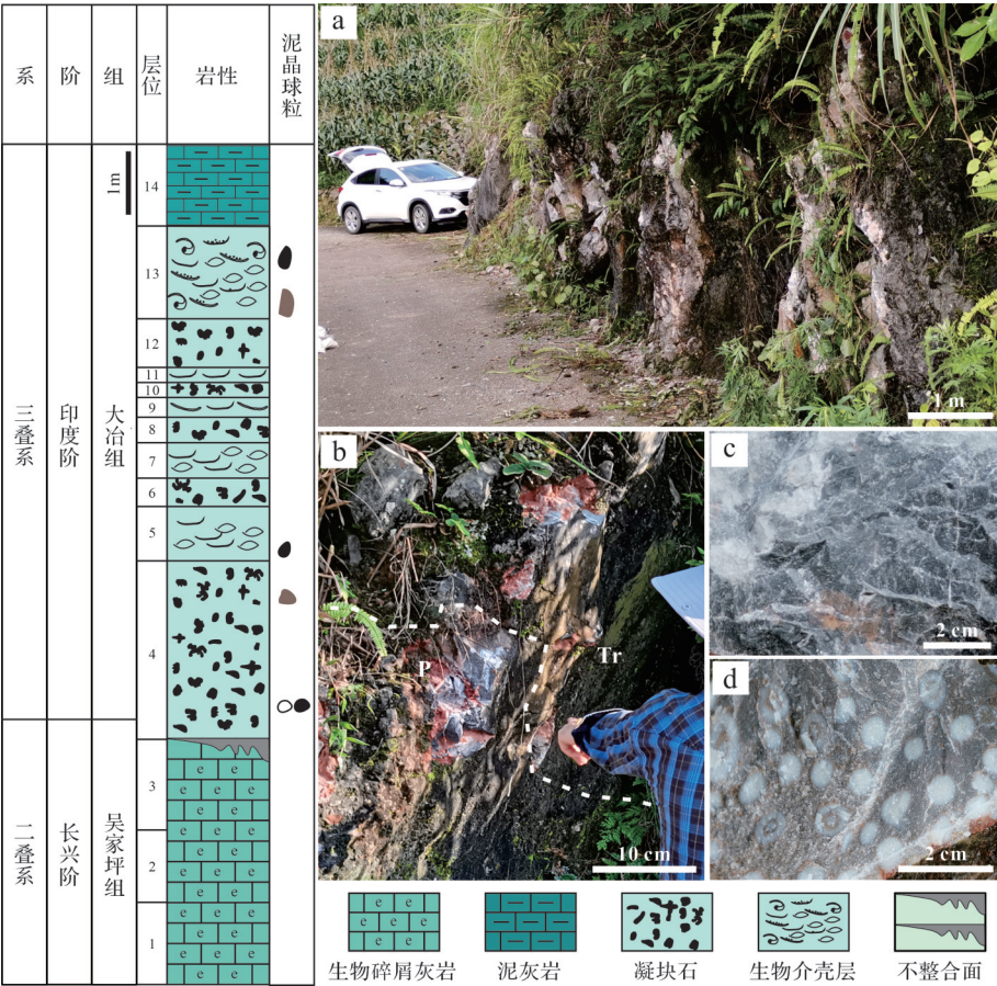
图2 田湾剖面微生物岩序列的岩性柱状图以及典型岩性类型的野外露头 (a)田湾剖面野外露头照片,主要显示微生物岩区段;(b)田湾剖面P—Tr界线处露头照片;(c)大冶组微生物岩中凝块石的野外照片;(d)吴家坪组含珊瑚的生物碎屑灰岩野外照片
