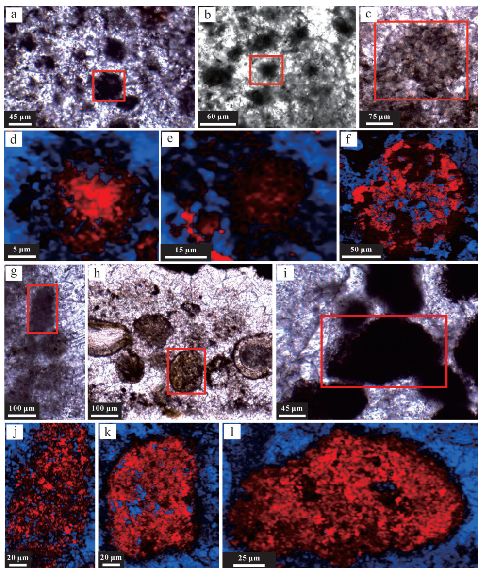
图 11 不同类型有机质球粒结构的拉曼光谱面分析结果
