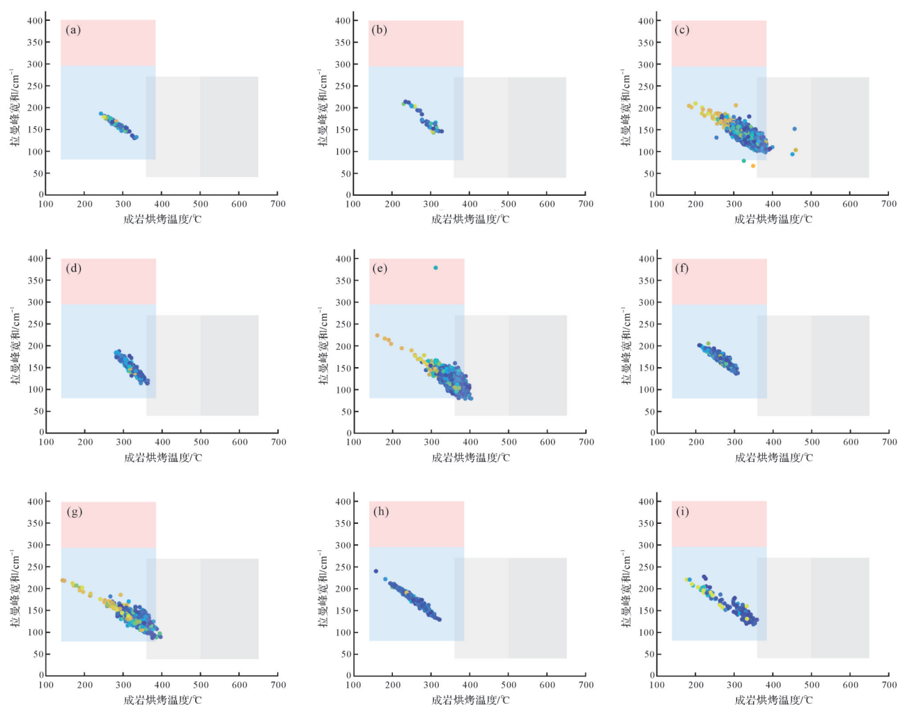
图 13 不同类型球粒、生物化石和介壳碎片外部泥晶套的有机质石墨化程度分析
