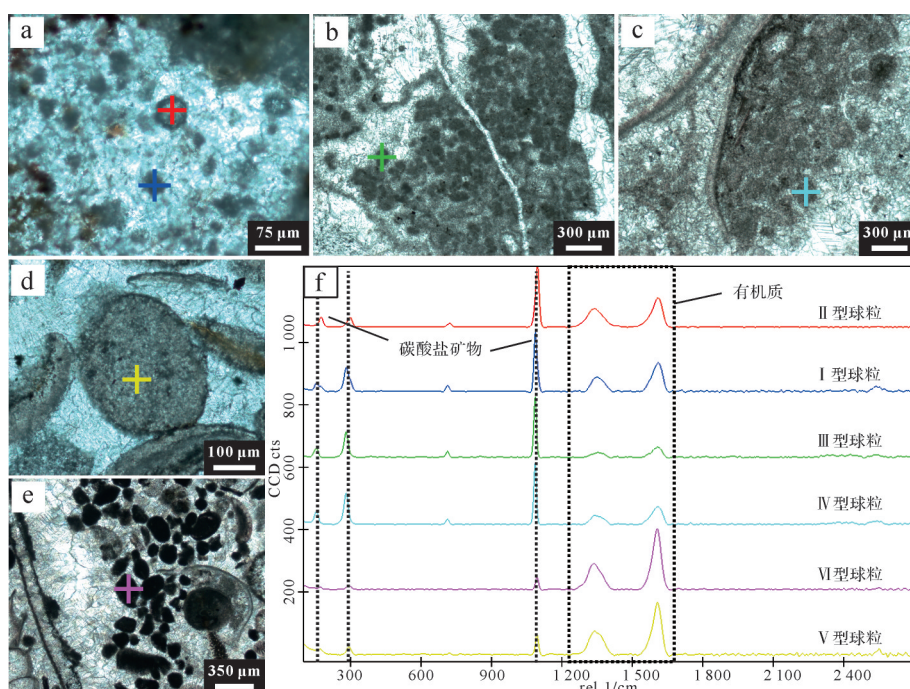
图10 不同类型有机质球粒结构的拉曼光谱点分析结果
