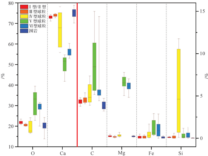
图9 不同球粒的能谱分析与元素组成对比
