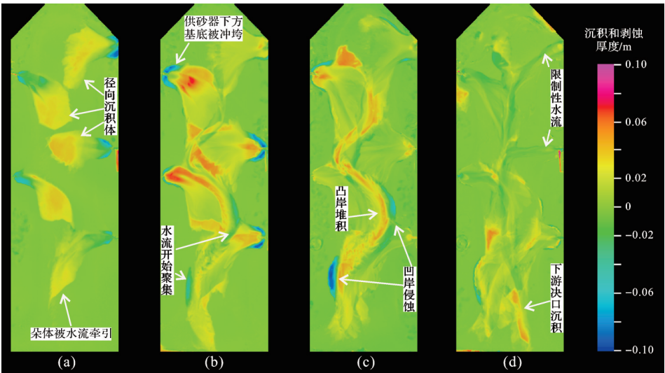
图4 实验过程中新增沉积体以及被剥蚀位置
