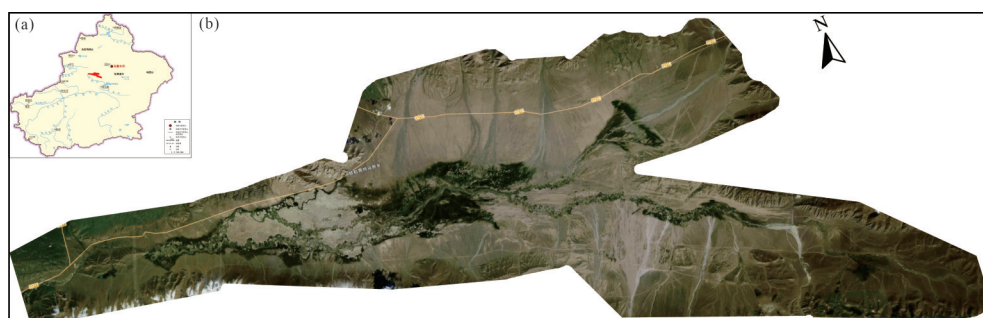
图7 小尤尔都斯盆地示意图
