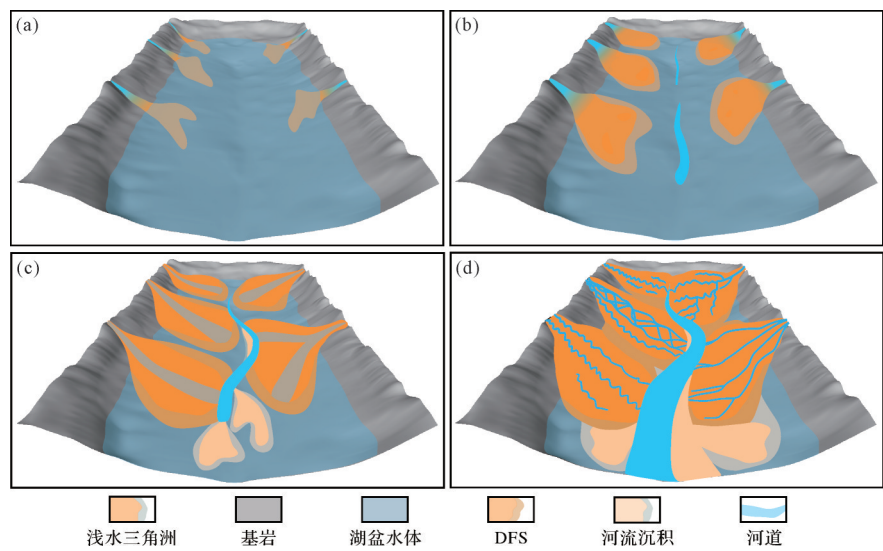
图9 狭长浅水湖盆DFS平面发育模式 (a)浅水三角洲发育期;(b)湖泊消亡期;(c)曲流河发育期;(d)曲流河决口期
