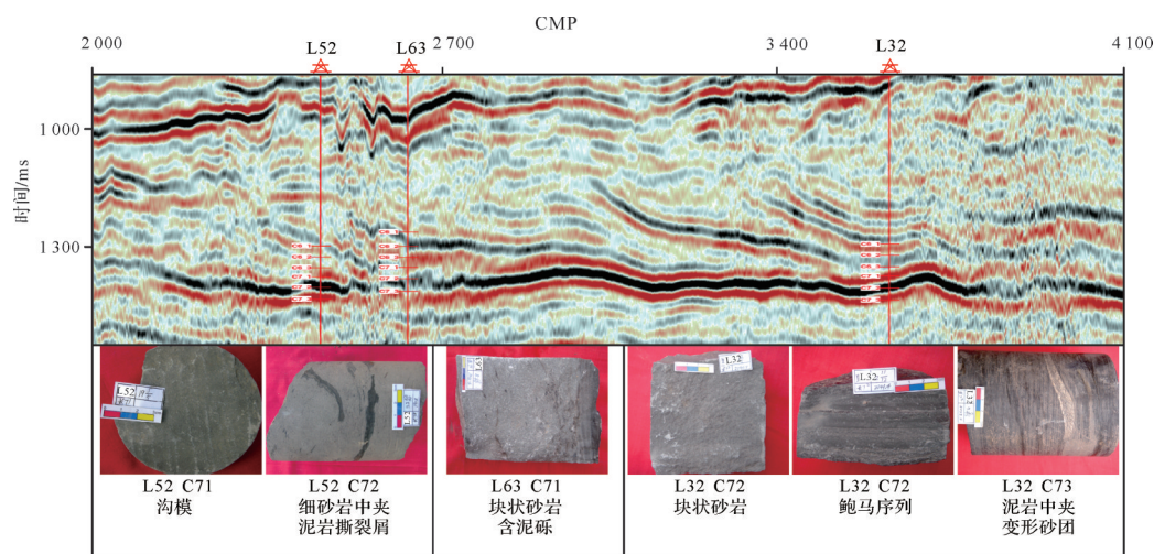
图16 过L52井—L63井—L32井地震剖面及岩心照片
