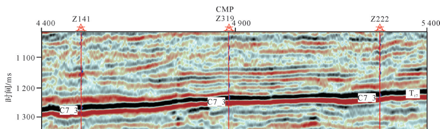
图5 陇东地区地震剖面
