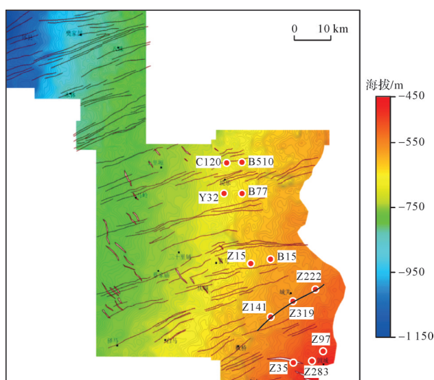
图4 陇东地区长 7 3 底现今构造图
