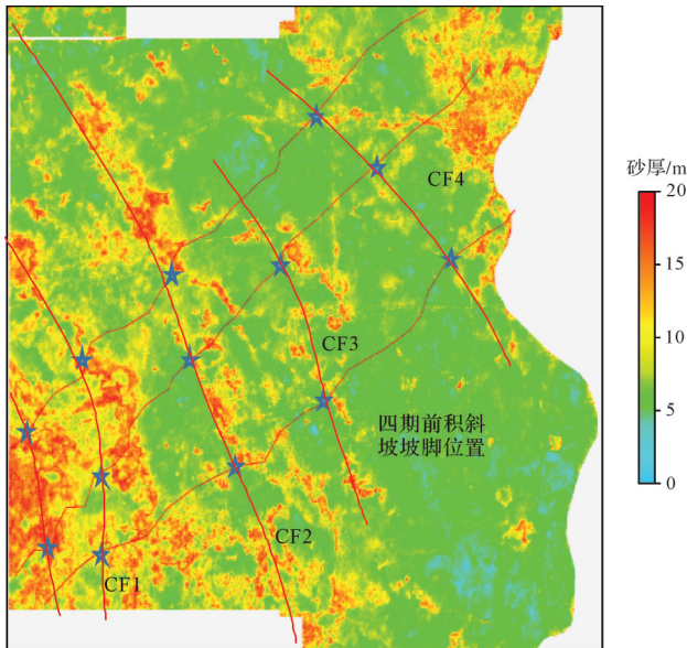
图9 长 7_3 亚段纹层型储层砂厚图
