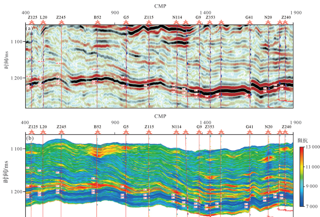
图10 陇东地区地震剖面(a)及纵波阻抗反演结果(b)
