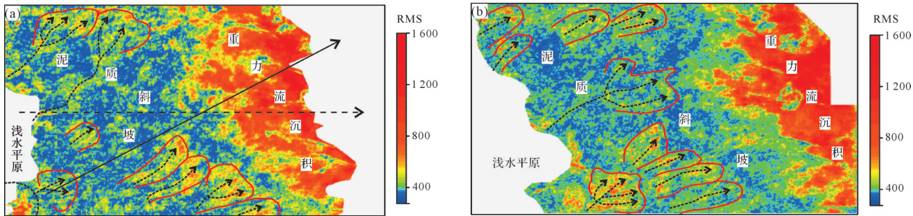
图 12 地震均方根属性 (a)CF3_1沿层切片;(b)CF3_2沿层切片 Fig.12 Root mean square (RMS) amplitude attribute of seismic data (a) CF3_1;(b) CF3_2
