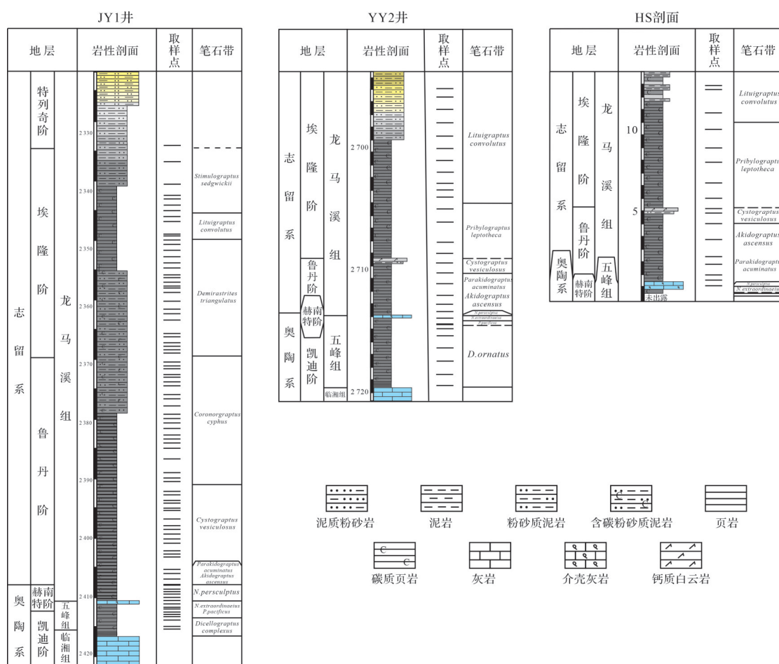
图2 川东与鄂西地区研究剖面五峰组—龙马溪组地层序列与样品位置
