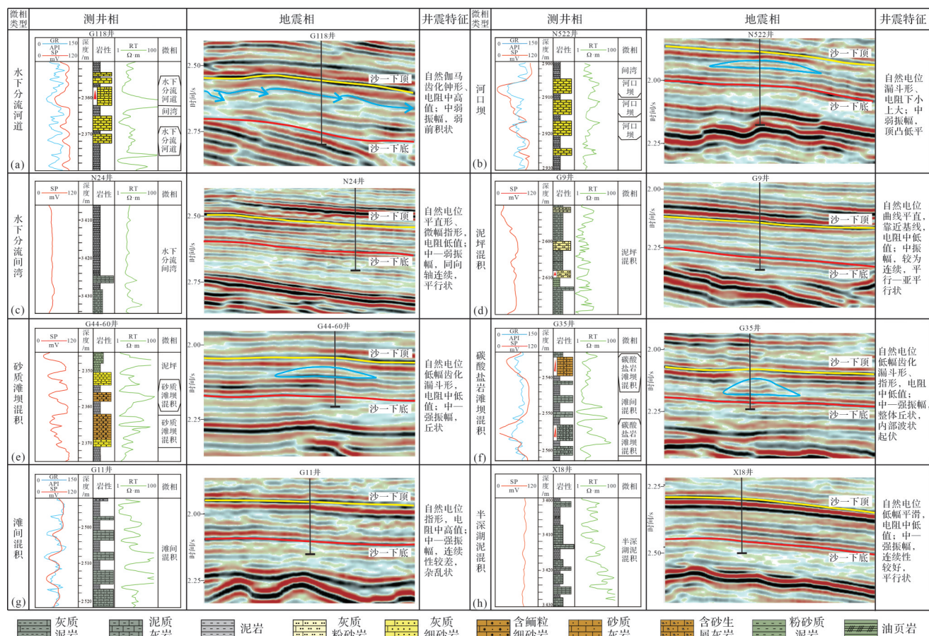
图4 蠡县斜坡沙一下亚段混合沉积不同微相井震特征
