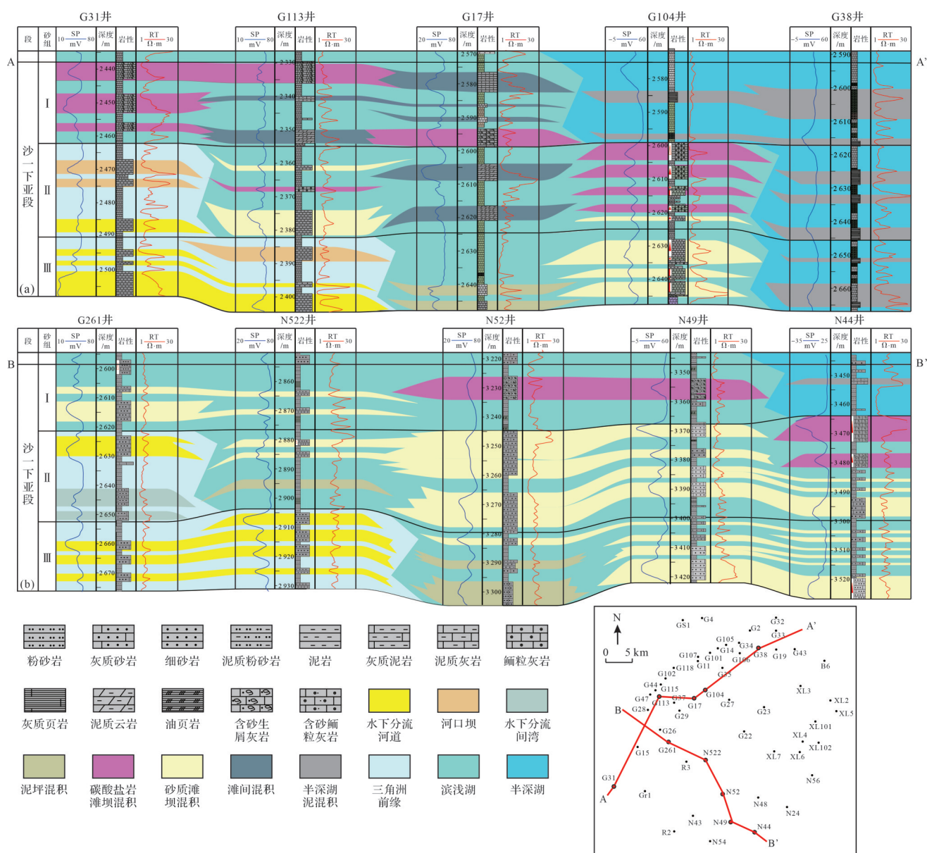
图5 蠡县斜坡沙一下亚段混合沉积连井相剖面
