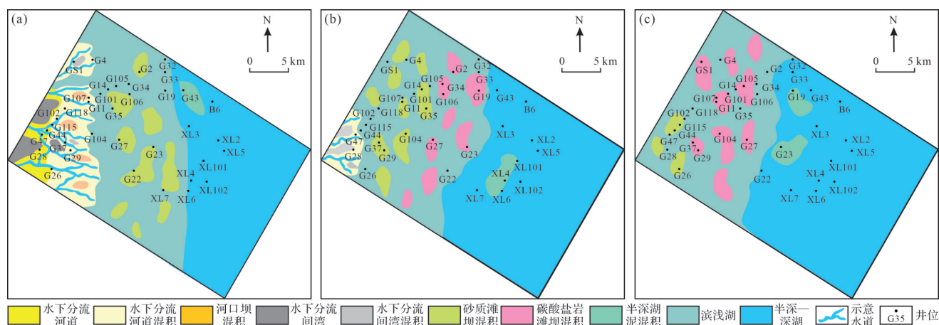
图6 蠡县斜坡沙一下亚段混合沉积微相特征 (a)Ⅲ砂组沉积微相;(b)Ⅱ砂组沉积微相;(c)Ⅰ砂组沉积微相
