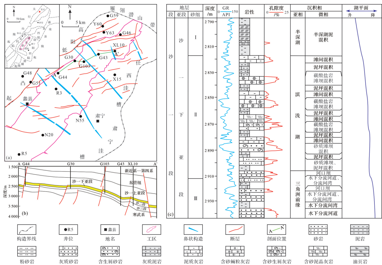
图1 蠡县斜坡工区概况 (a)研究区位置图;(b)剖面位置图;(c)沙一下亚段地层综合柱状图 Fig.1 Overview of the Lixian slope
