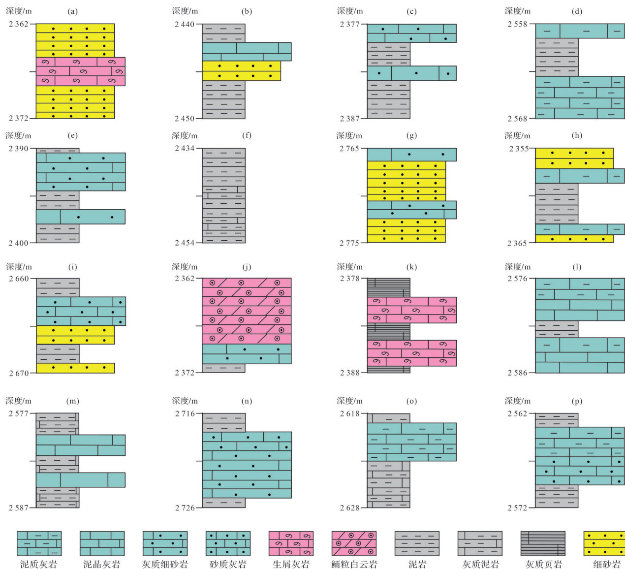
图3 蠡县斜坡沙一下亚段混积层系类型
