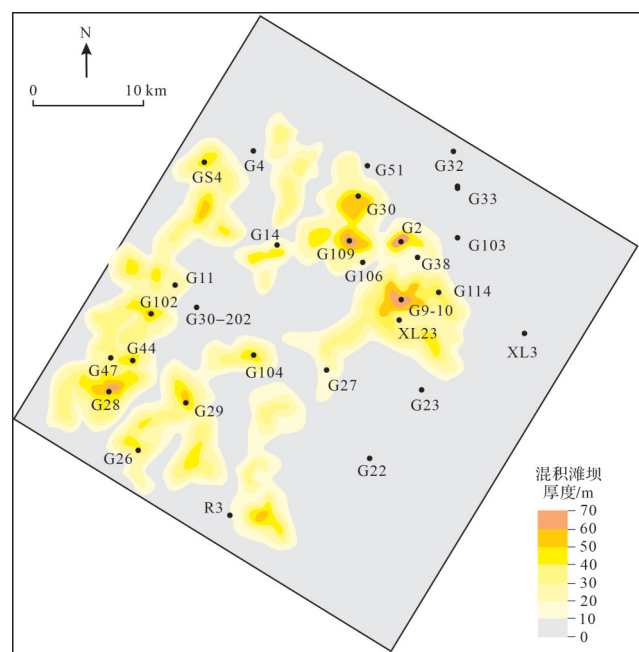
图10 蠡县斜坡沙一下亚段混合沉积有利储层分布预测
