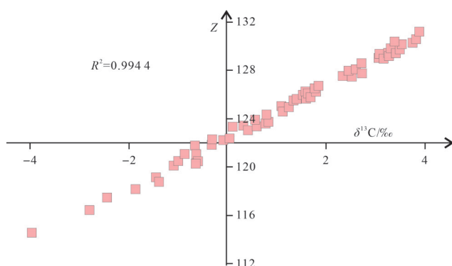
图8 四川盆地东部高台组碳酸盐岩—蒸发岩 \delta^{13}\text{C} -Z值关系图
