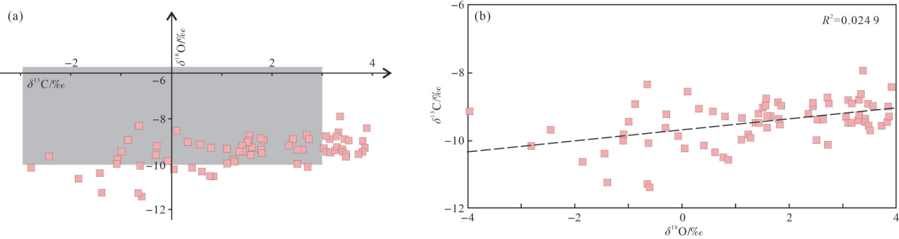
图7 四川盆地东部高台组碳酸盐岩—蒸发岩碳氧同位素值关系图
