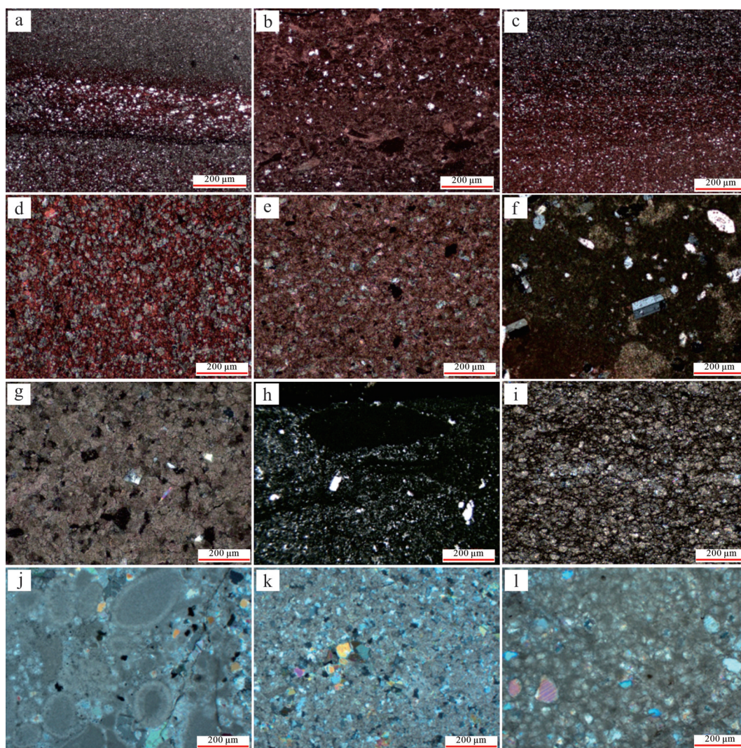
图2 碳酸盐岩—蒸发岩共生体系白云岩镜下特征
