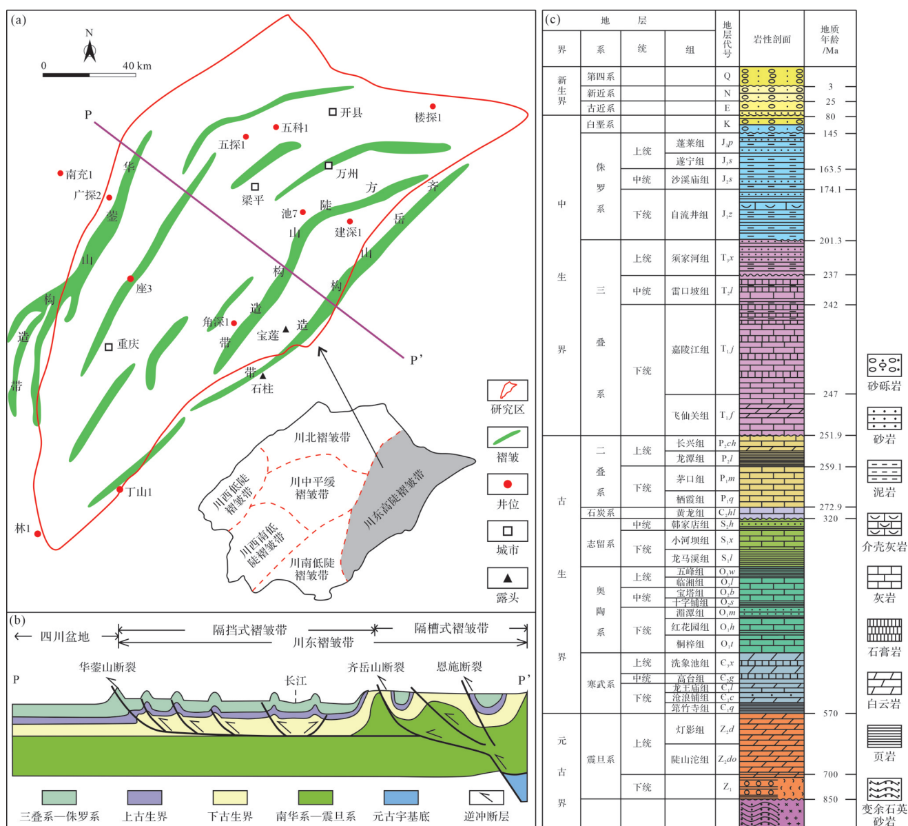
图1 (a) 研究区构造分区图; (b) 研究区构造剖面图 (Yan et al. , 2003; 胡召齐等, 2009);
