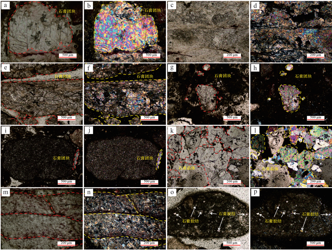
图3 碳酸盐岩—蒸发岩共生体系蒸发岩镜下特征 (a,b)石膏岩,楼探1井,5 965.00 m;(c,d)石膏岩,楼探1井,5 595.00 m;(e,f)石膏岩,楼探1井,6 763.00 m;(g,h)石膏岩,磨空严重,楼探1井,5 670.00 m;(i,j)含石膏泥晶白云岩,仅剩一颗岩屑,楼探1井,5 665.00 m;(k,l)石膏质泥晶白云岩,部分较大的石膏晶体间见晶间孔,也见较大晶体的白云石,楼探1井,5 602.00 m;(m,n)含白云石膏岩/石膏岩,楼探1井,6 558.00 m;(o,p)含石膏泥晶白云岩,楼探1井,6 435.00 m
