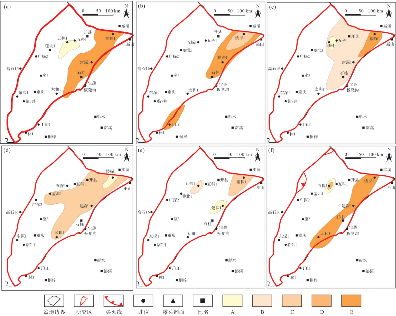
图6 碳酸盐岩—蒸发岩共生体系平面特征
