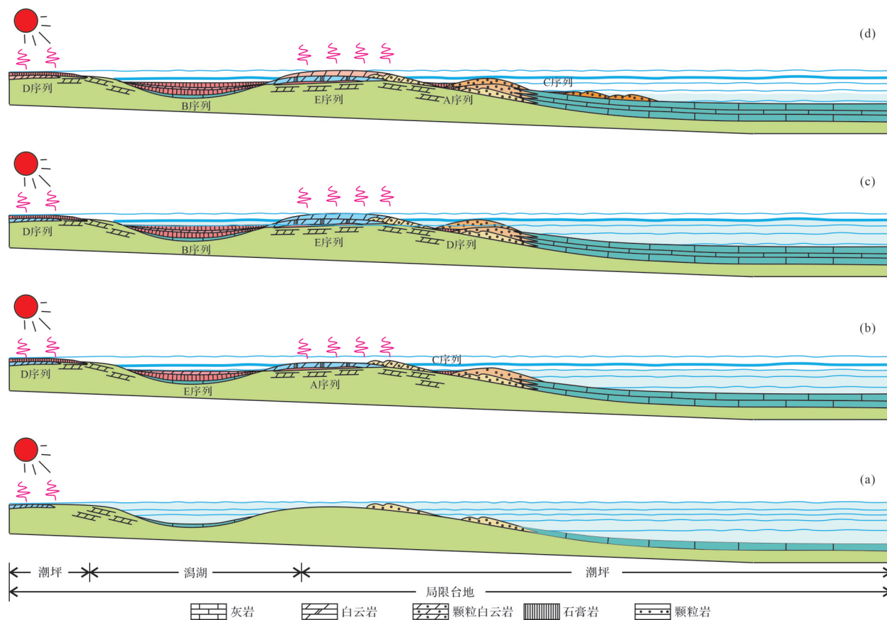
图12 四川盆地东部高台组碳酸盐岩—蒸发岩共生体系沉积机理
