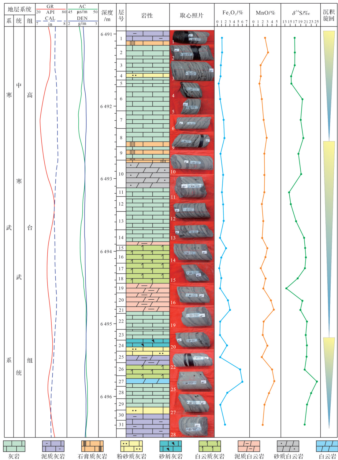
图9 四川盆地东部高台组楼探1井Fe、Mn含量及S同位素组成(δ 34 S)特征
