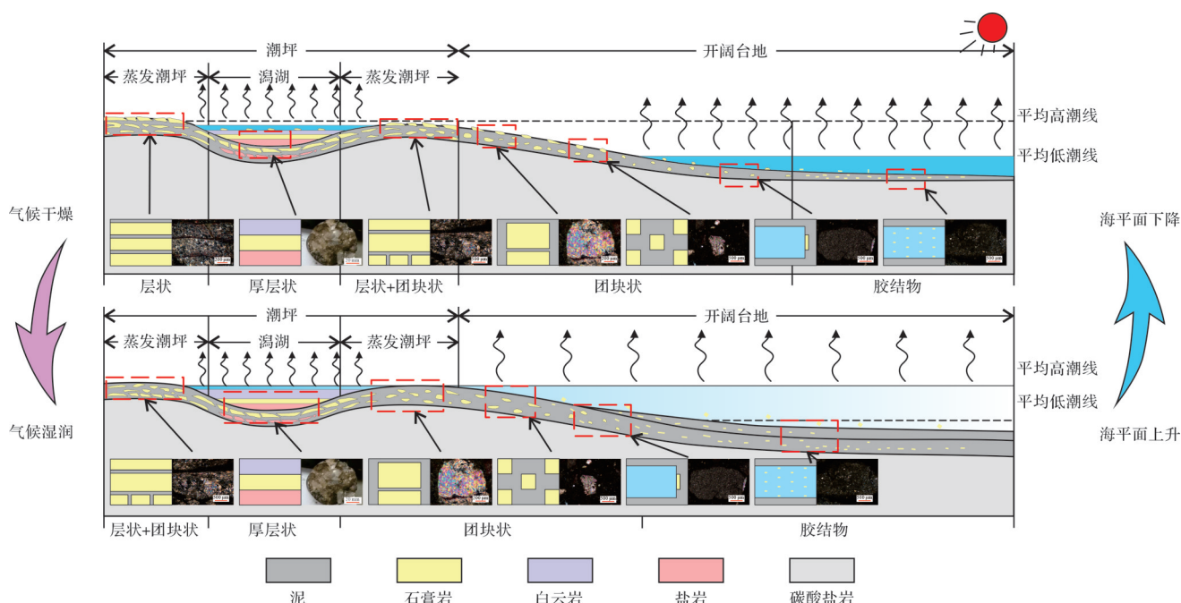
图13 四川盆地东部高台组碳酸盐岩—蒸发岩共生体系沉积演化模式
