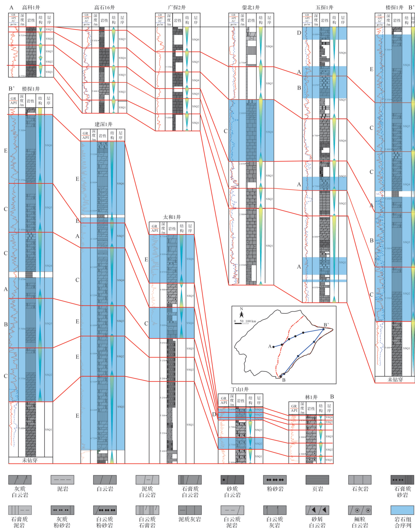
图5 碳酸盐岩—蒸发岩共生体系连井特征
