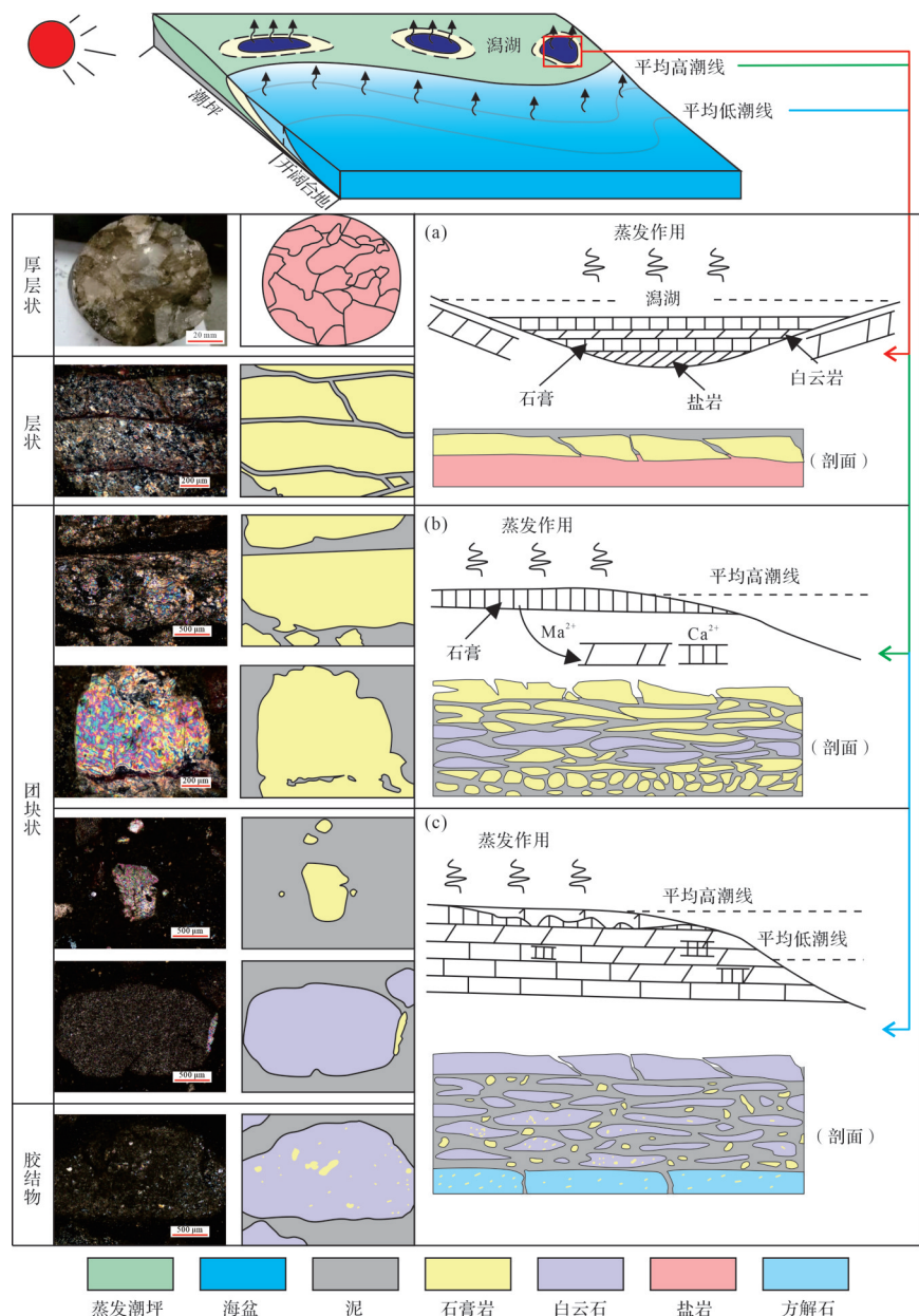
图 11 四川盆地东部高台组碳酸盐岩—蒸发岩共生体系沉积过程
