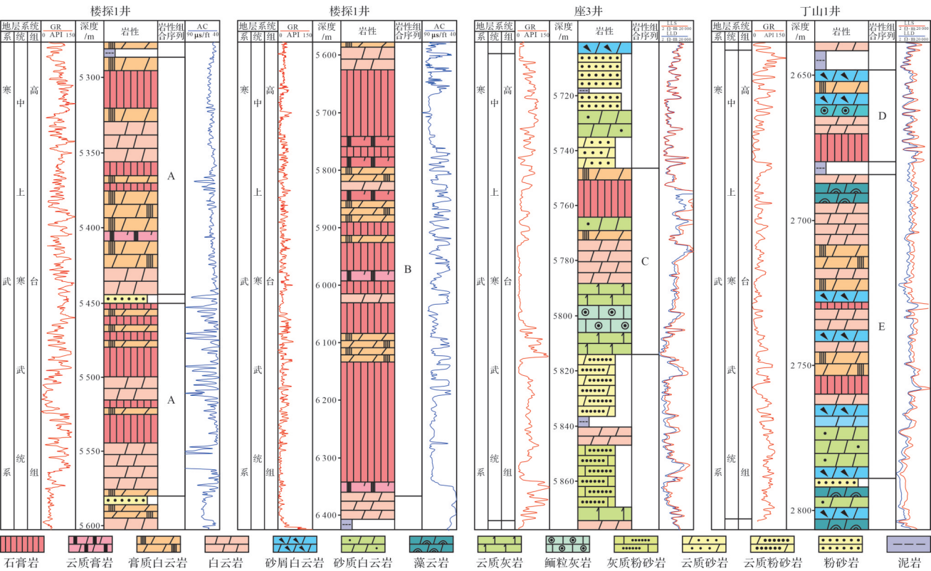
图4 碳酸盐岩—蒸发岩共生体系岩石组合序列
