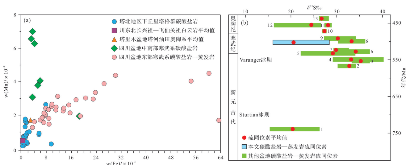
图10 四川盆地东部与其他盆地 Fe、Mn 含量及 S 同位素组成 ( \delta^{34}\text{S} ) 特征
