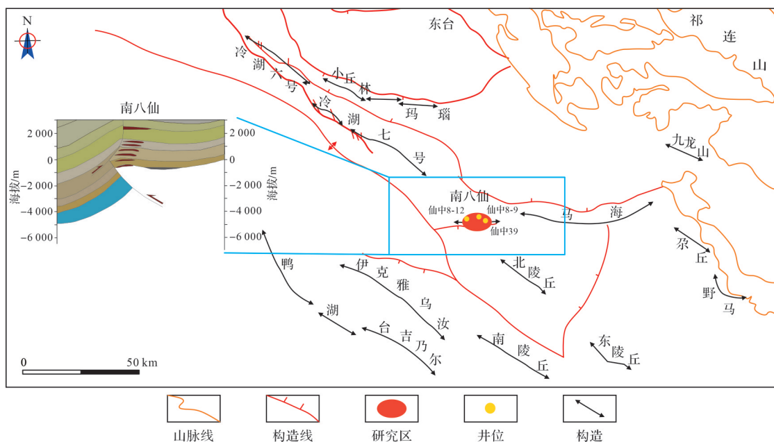
图1 南八仙油气田地质概况
