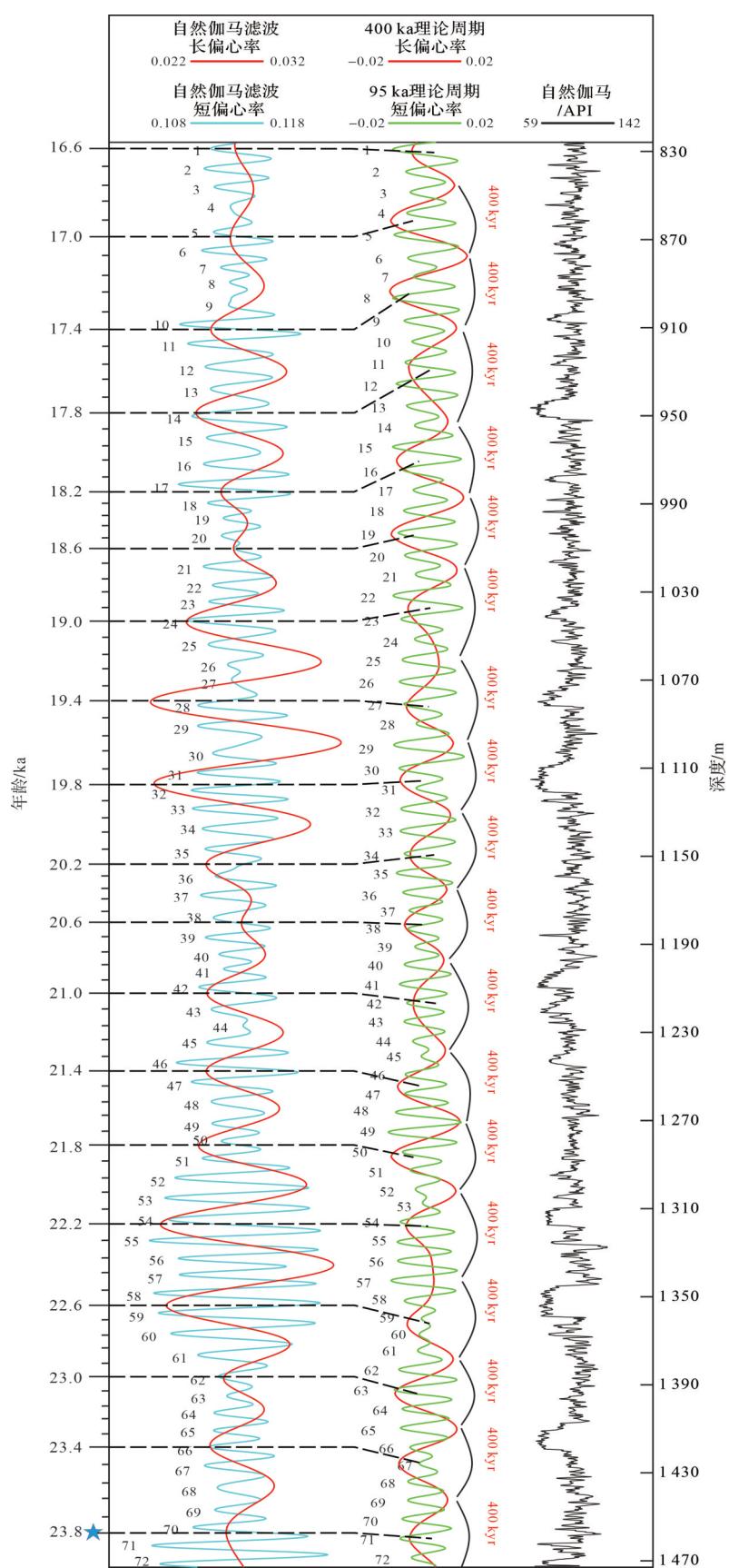
图7 仙中39井天文年代标尺
