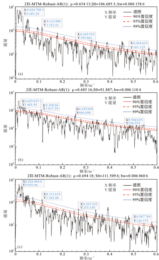
图5 柴达木盆地南八仙油气田下油砂山组频谱分析图 (a)仙中39井;(b)仙中8-12井;(c)仙中8-9井
