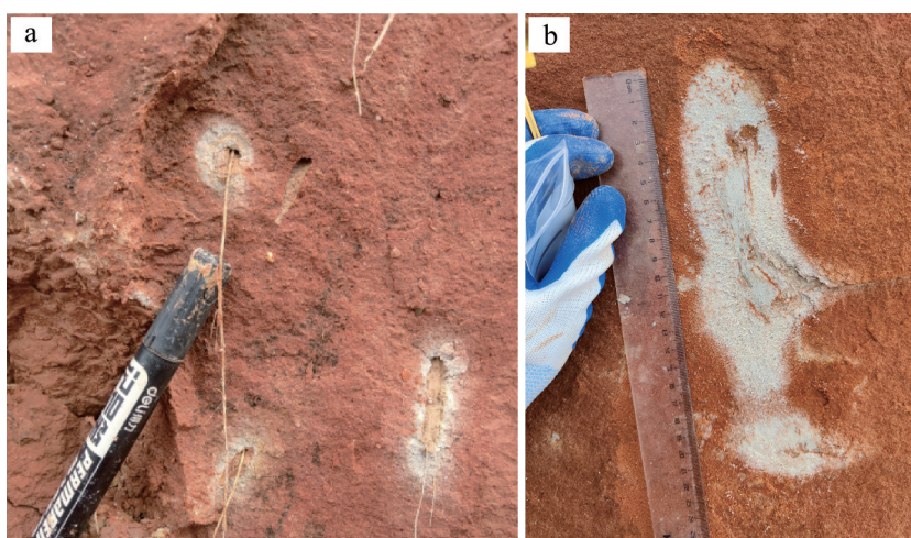
图2 红色砂岩(基岩)中的网纹 Fig.2 Reticulation in red sandstone (bedrock)
