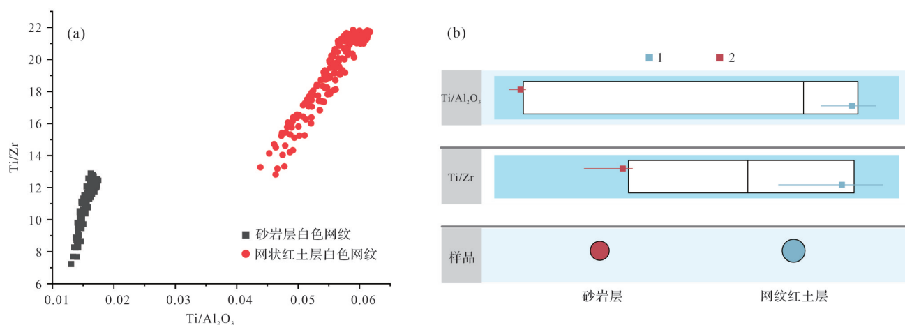
图5 稳定元素比值与聚类比较
