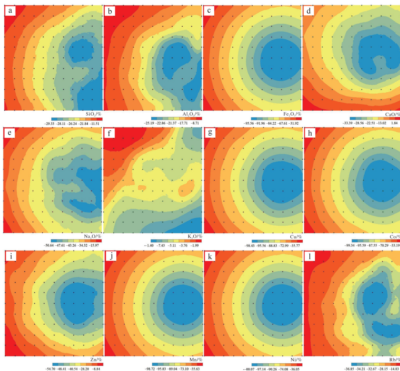
图7 砂岩白色网纹微区元素迁移分布
