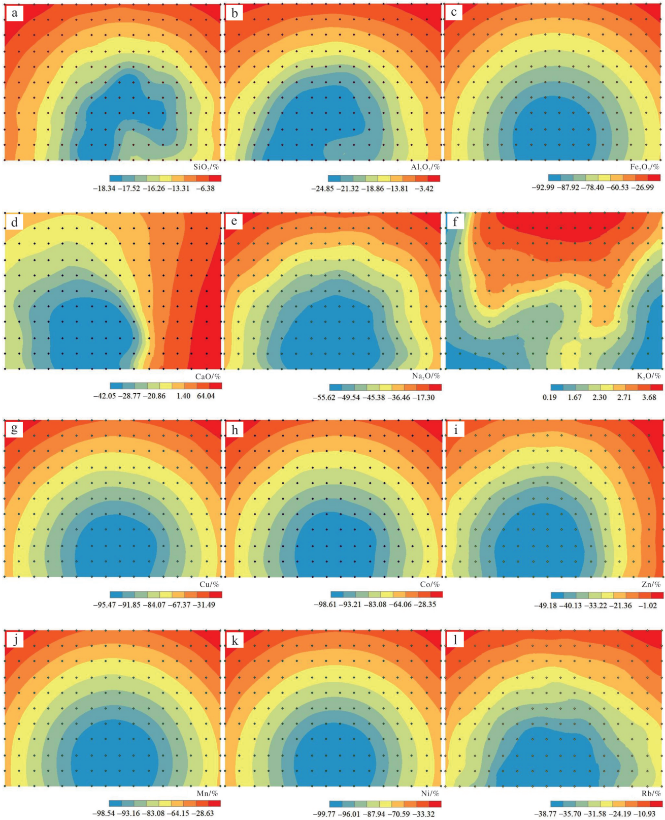
图6 网纹红土层白色网纹微区元素迁移分布
