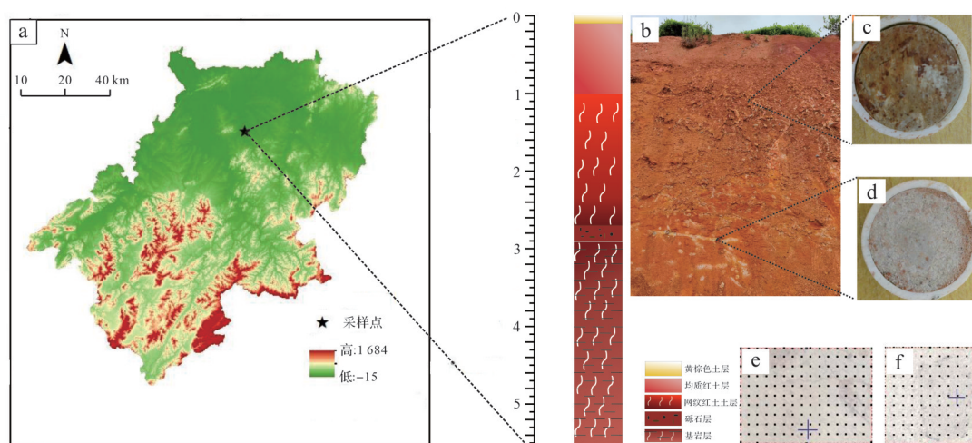
图1 观测点位置示意图
