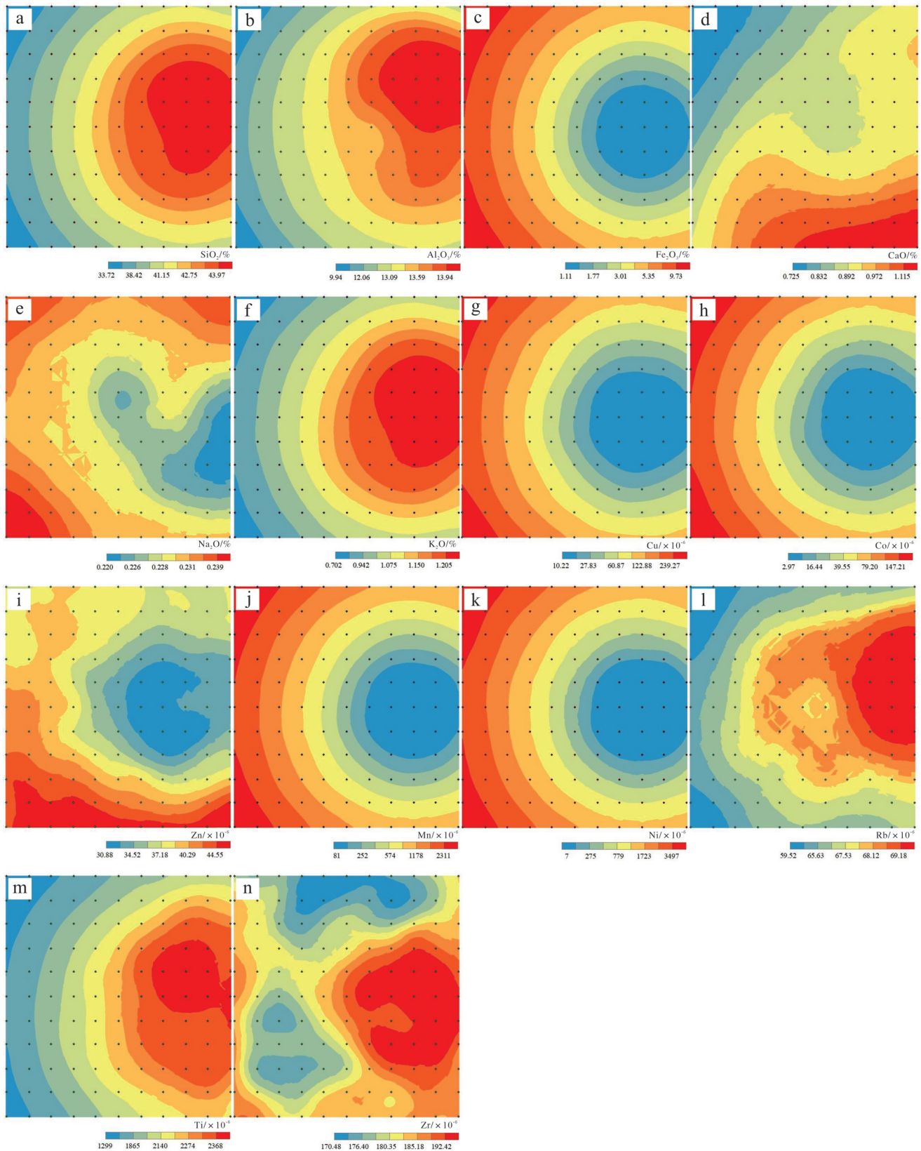
图4 砂岩白色网纹微区元素变化
