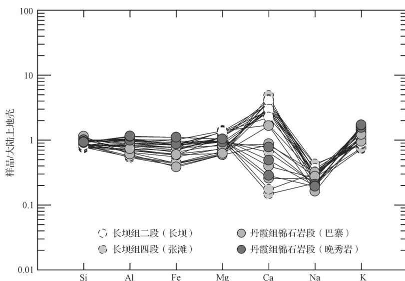
图6 丹霞盆地上白垩统长坝组—丹霞组细粒碎屑岩大陆上地壳标准化曲线
