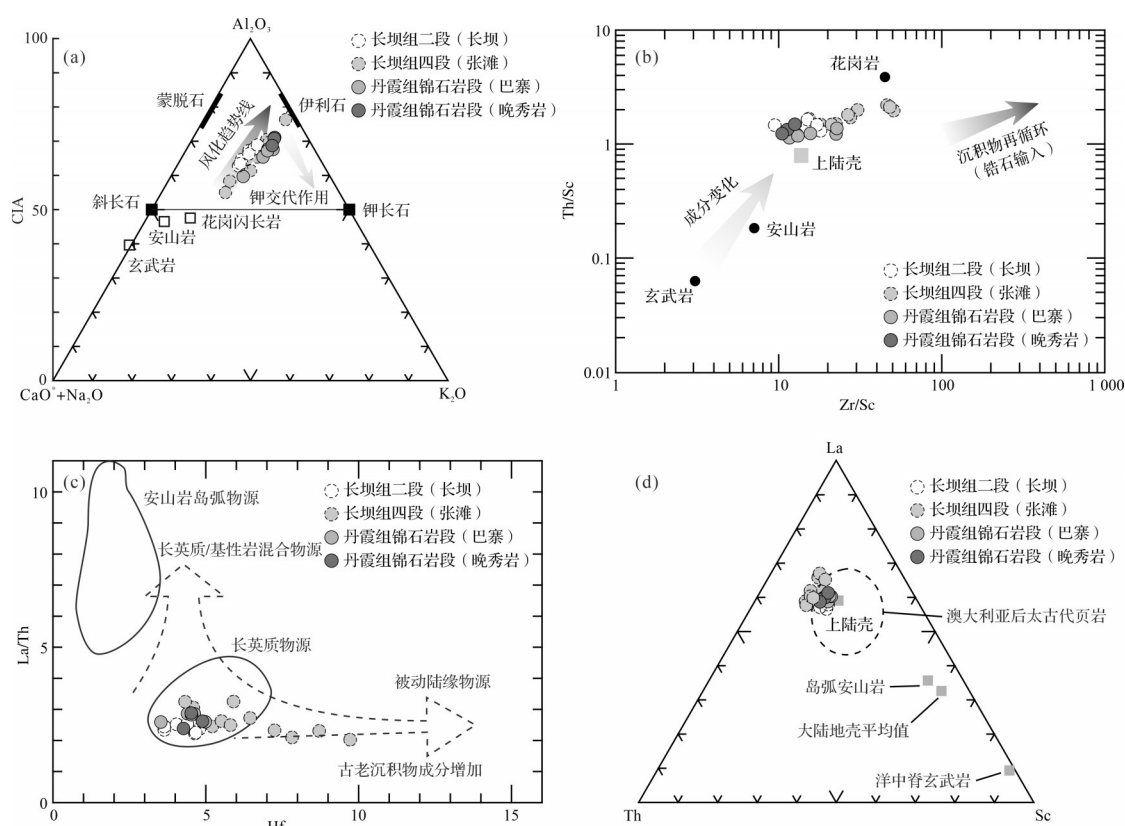
图 12 (a) 丹霞盆地上白垩统长坝组—丹霞组细粒碎屑岩化学蚀变指数 CIA 及 Al_2O_3 - CaO+Na_2O - K_2O 图解 (Nesbitt and Young, 1984; McLennan et al. , 1993; Fedo et al. , 1995), 其中 CaO^* 为硅酸盐矿物中的 CaO , 计算方法见 McLennan (1993); (b) Th/Sc-Zr/Sc 图解 (底图据 McLennan et al. , 1993), 黑色圆点代表花岗岩、安山岩和玄武岩的平均成分 (数据来自 Condie, 1993), 灰色方块代表了大陆上地壳的平均成分 (Rudnick and Gao, 2003; Hu and Gao, 2008), 左侧箭头指示成分差异, 右侧箭头代表沉积物再循环; (c) La/Th-Hf 图解 (底图据 Floyd and Leveridge, 1987); (d) La-Th-Sc 三角图解, 潜在物源数据来自 McLennan and Taylor (1984)
