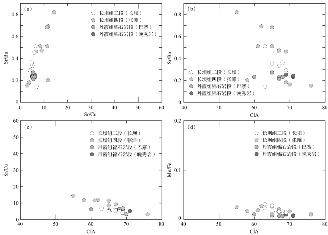
图 14 Sr/Ba、Sr/Cu、Mn/Fe 及 CIA 关系图解 Fig.14 Relationships between Sr/Ba, Sr/Cu, Mn/Fe and CIA
