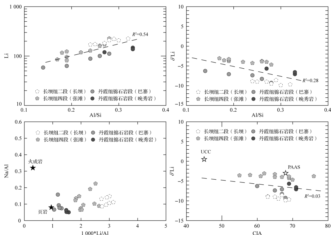
图13 (a,b) Al/Si 与 Li 含量以及 Li 同位素关系图解; (c) Li/Al 与 Na/Al 比值的关系图; 黑色五角星代表两个源岩端元, 火成岩和页岩端元数据来自 Dellinger et al. , (2014); (d) CIA 与 Li 同位素的相关性, 上地壳 (UCC) 和澳大利亚后太古代页岩 (PAAS) 值来自 Taylor and McLennan (1985) 及 Mude et al. (2019)
