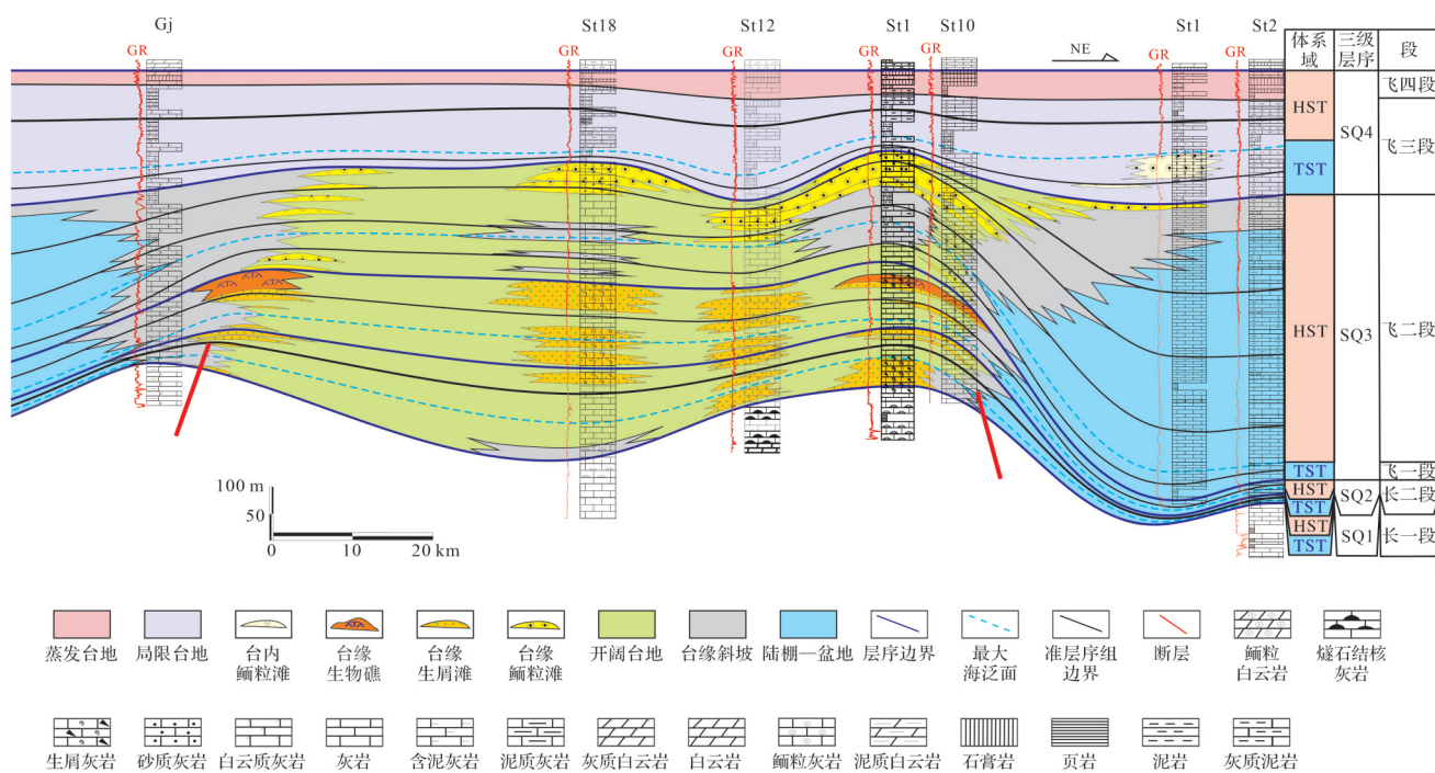
图7 过Gj井—St2井长兴组—飞仙关组层序地层和沉积相对比剖面图
