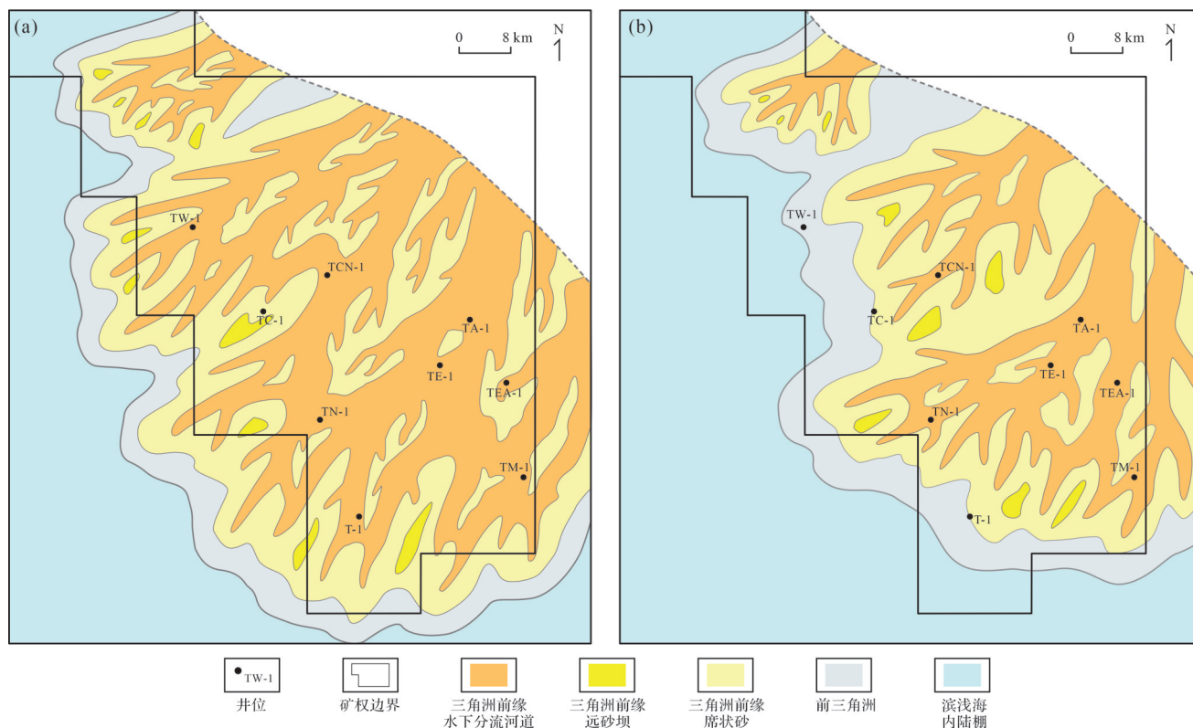
图4 Trakes斜坡上白垩统Donga组DS1段(a)和DS3段(b)沉积相图
