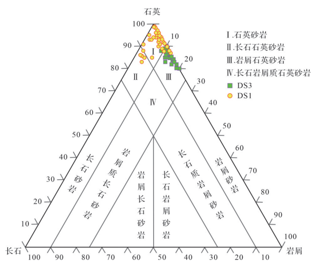
图5 Trakes斜坡上白垩统Donga组砂岩类型三角图
