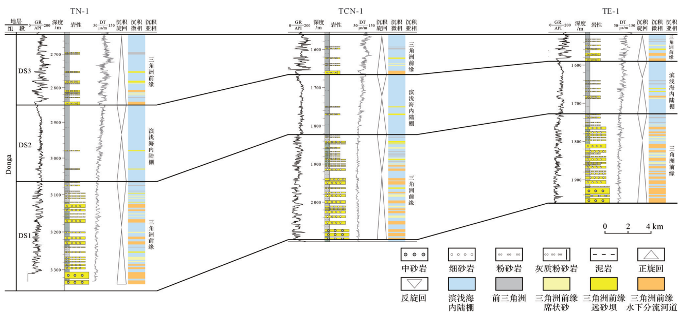
图3 Trakes斜坡上白垩统Donga组连井地层对比
