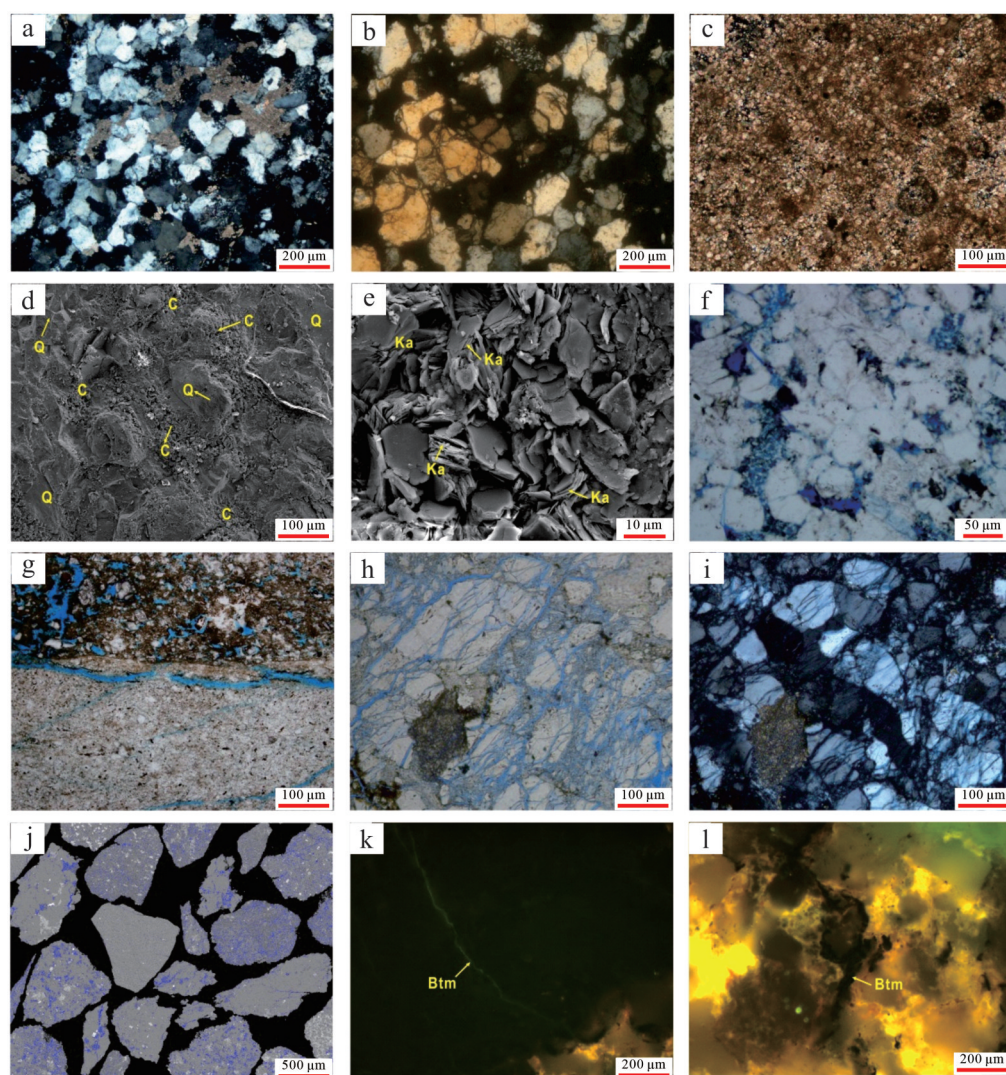
图6 Trakes斜坡上白垩统Donga组储层岩石薄片、扫描电镜和背散射物性分析图
