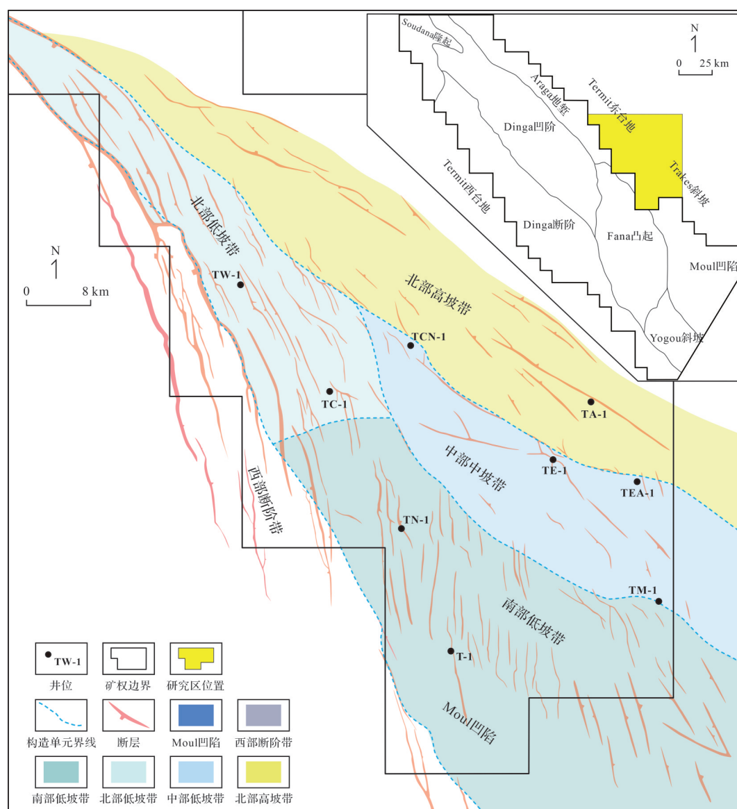
图1 Termit盆地Trakes斜坡区域位置、构造单元划分(据刘邦等,2012b修改)及取样井位图
