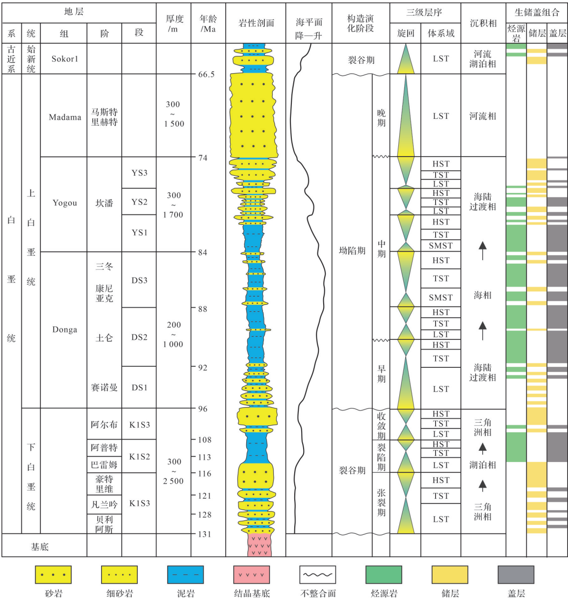
图2 Termit盆地白垩系综合柱状图(据 Genik, 1993 修改)
