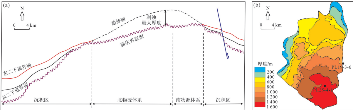
图6 渤南低凸起中生界剥蚀厚度计算方法与厚度分布 (a)物源区地层剥蚀厚度计算方法;(b)剥蚀厚度平面分布
