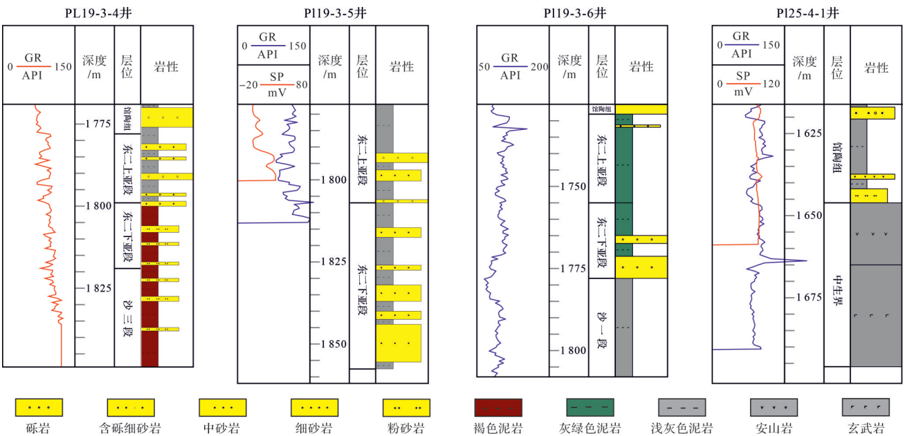
图5 渤南低凸起东二下段钻井与地层发育特征
