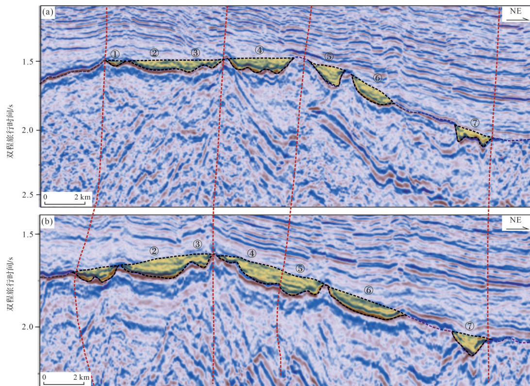
图7 渤南低凸起古沟谷特征
