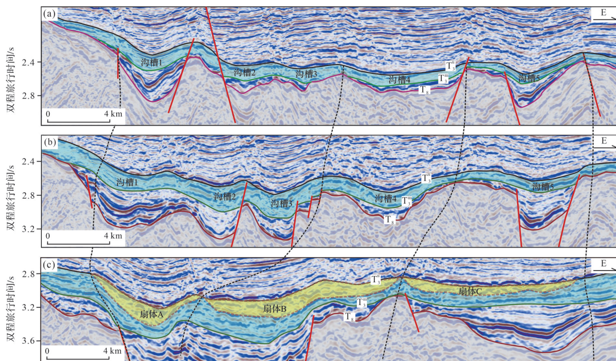
图9 渤中凹陷东南斜坡带古沟槽特征
