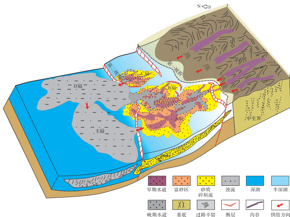
图 12 东二下层序湖底扇充填演化模式
