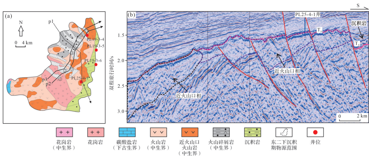
图4 渤南低凸起东段东二下时期物源体系特征(剖面位置见图P1)
