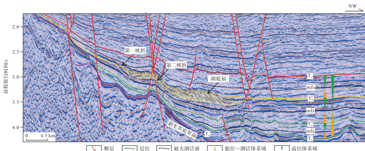
图2 渤中凹陷东南斜坡带东营组层序地层特征(剖面位置见图1中P1)
