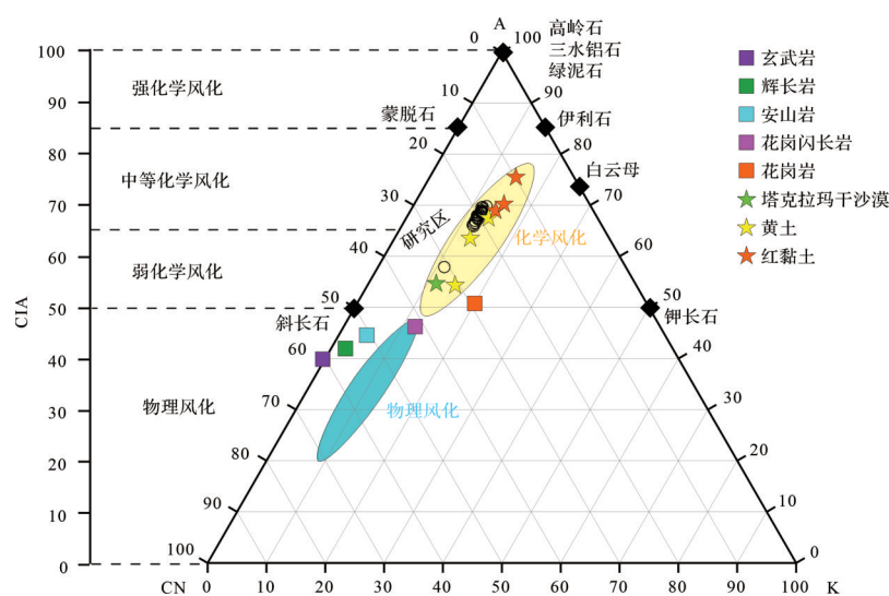
图4 研究区沉积物 A-CN-K 三角图解 (底图据 Zhang et al. , 2020; 丁雪等, 2023 修改)
