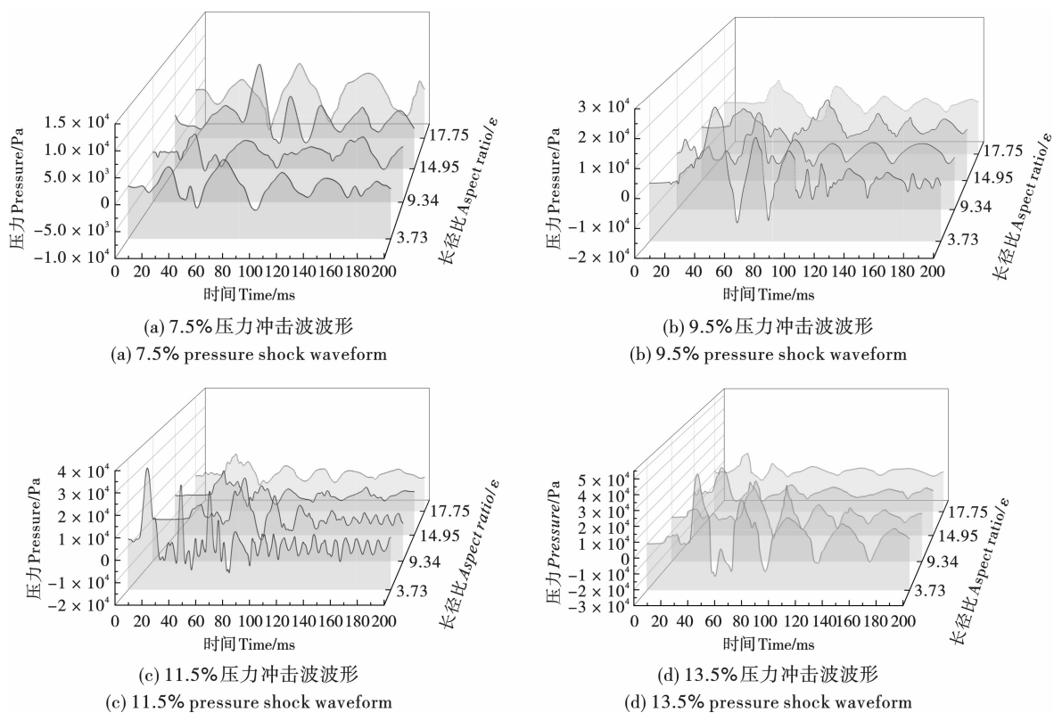
图3 压力波形曲线图
