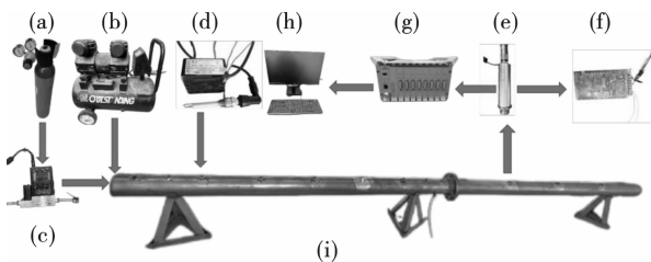
(a) 甲烷气瓶 (b) 空压机 (c) 流量计 (a) Methane cylinders (b) Air compressor (c) Flowmeter (d) 点火器 (e) 压力传感器 (f) 稳压器 (d) Igniter (e) Pressure sensors (f) Voltage regulators (g) 采集仪 (h) 电脑 (i) 试验管道 (g) Collector (h) Computer (i) Pilot pipelines
