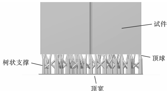
图 2 树状支撑图
