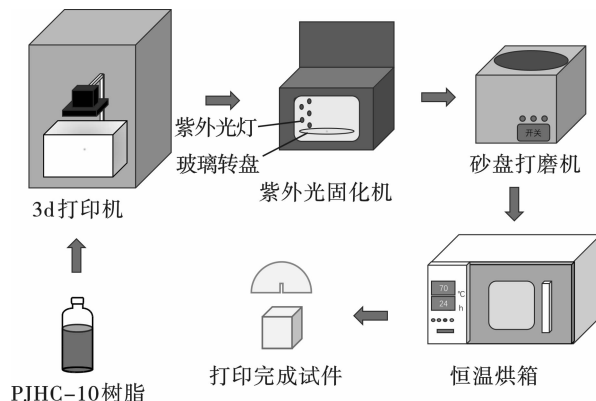
图 3 打印流程图
