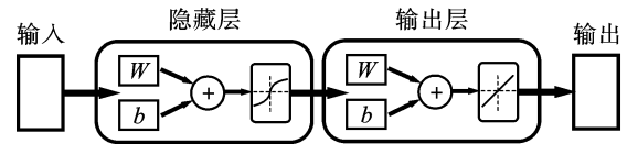
图 6 ANN 模型结构示意图 (注:修正权重参数 w 和偏置参数 b ) Fig. 6 Structure diagram of ANN model
