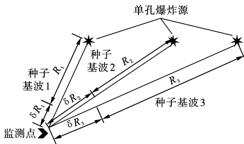
图 5 种子基波选取示意图 Fig. 5 Schematic diagram of seed fundamental wave selection
