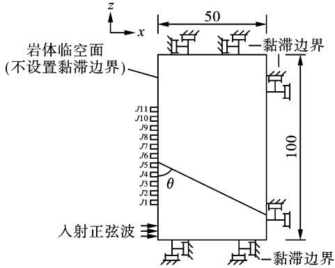
图 4 不同倾角结构面计算模型(单位:m)
