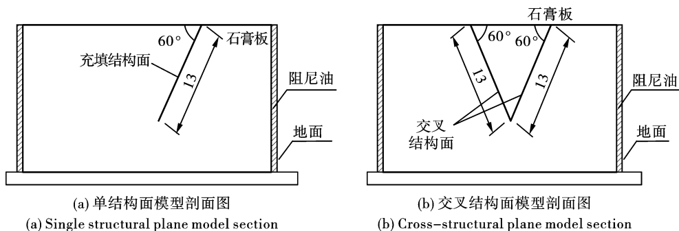
图 1 结构面模型示意图 Fig. 1 Structural plane model
