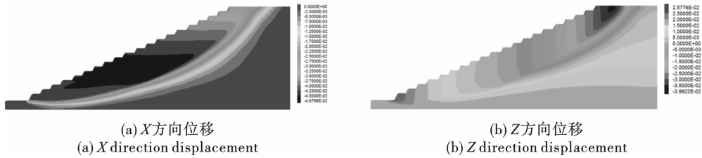
图 10 边坡折减条件下位移
