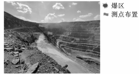
图3 爆破振动监测点布置
