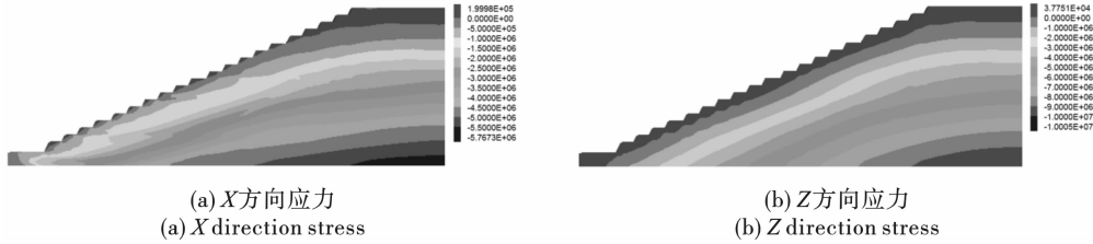
图 9 边坡折减条件下应力分布
