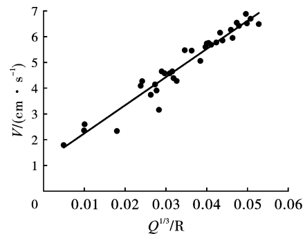
图5 爆破振动合速度回归曲线
