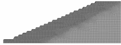
图6 边坡模型
