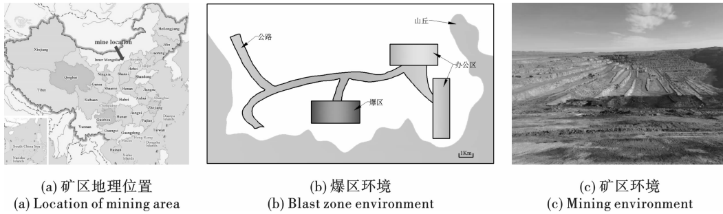
图1 矿区概况
