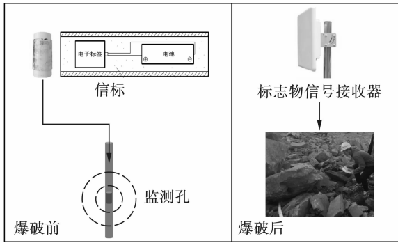
图2 信标系统 Fig.2 Beacon system
