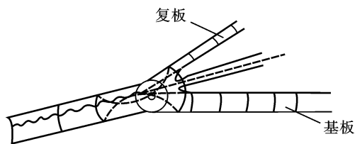
图8 碰撞应力波在基、复中传播的示意图
