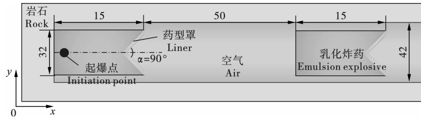
图3 炸药间隔50 cm时数值计算模型示意图(单位:cm)
