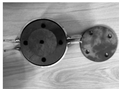
图2 钢制夹具
