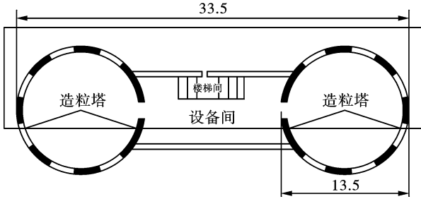
图 4 切口平面图(单位:m)
