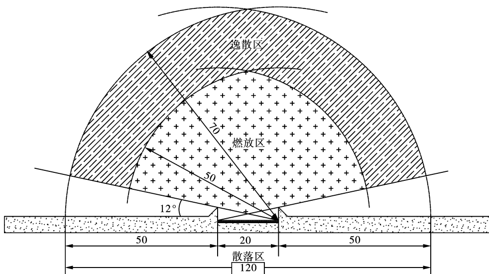
图 6 警戒区域界定图(单位:m)
